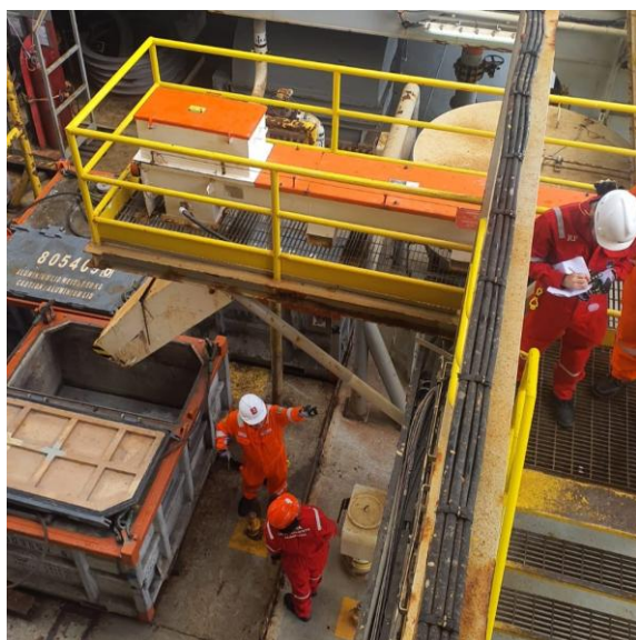
Fig. 11 - Sistema de recolhimento contingencial do cascalho
