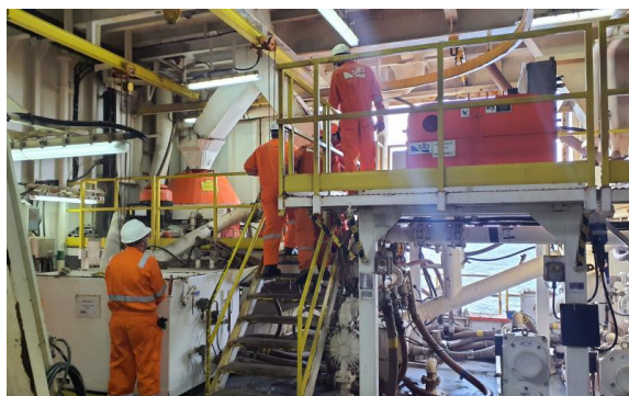
Fig. 7 - Sistema de secagem de cascalho
