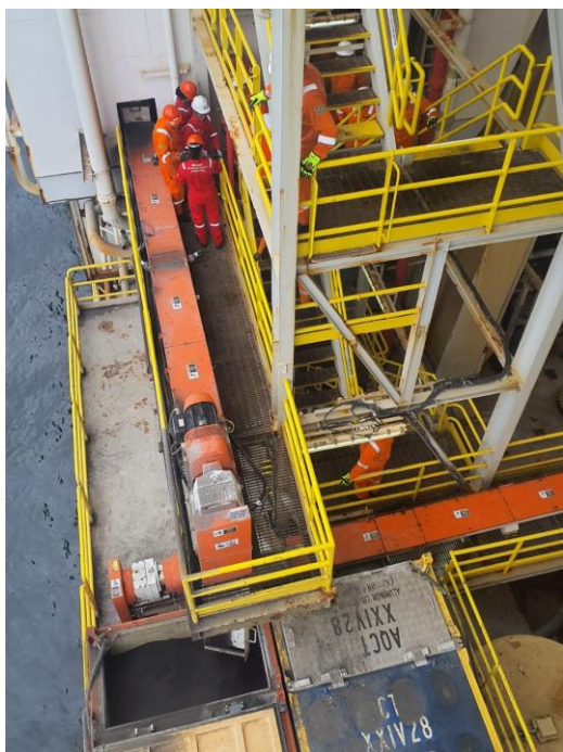
Fig. 9 - Sistema de recolhimento do cascalho das secadoras até o cutting box
