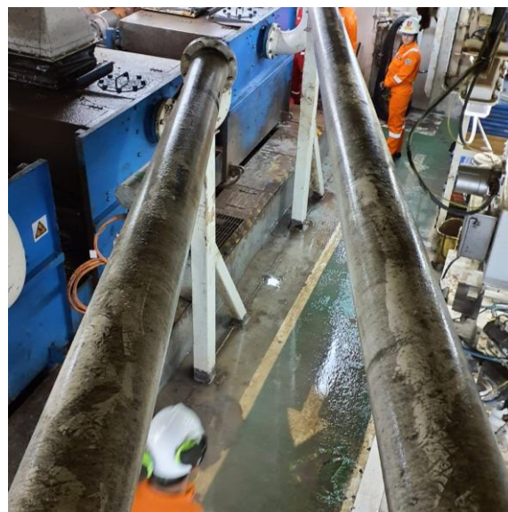
Fig. 4 - Rota de chegada do cascalho às peneiras
