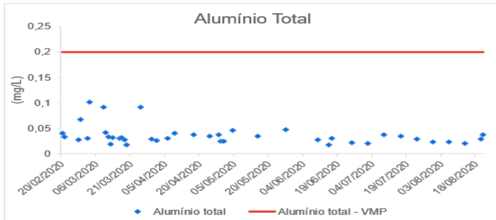
Figura 2: Monitoramento de Alumínio total (mg/L) na água tratada da ETA de Galileia
