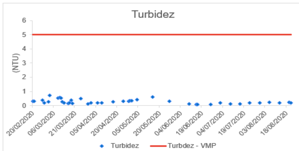
Figura 1: Monitoramento da Turbidez (NTU) na água tratada da ETA de Galileia
