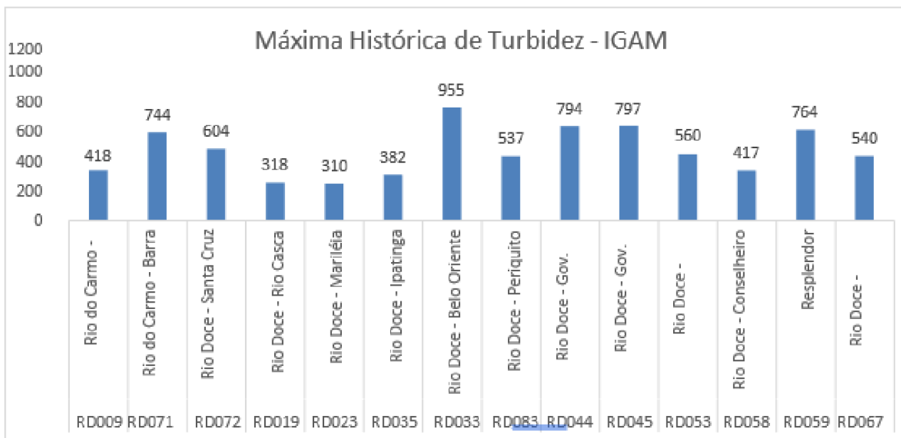
Figura 2: Valores máximos de turbidez – monitoramento do IGAM
