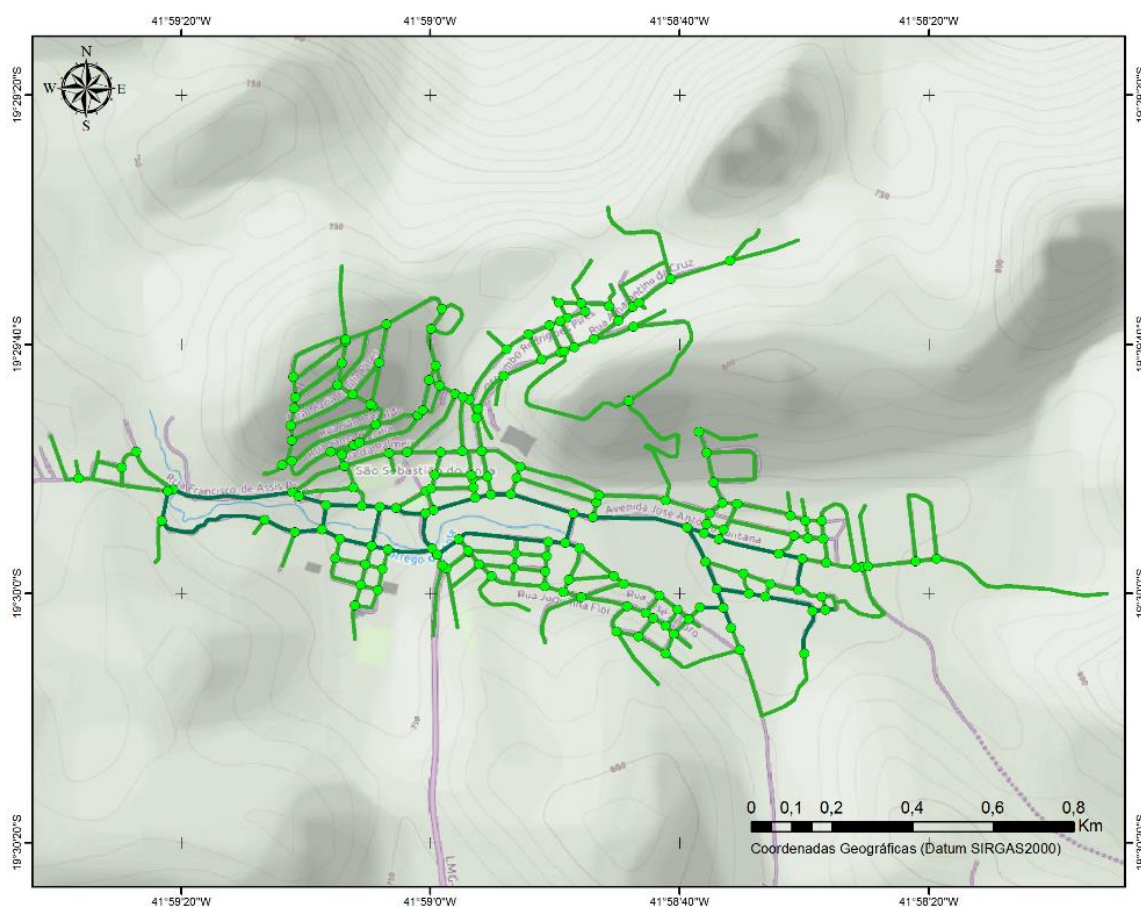
Figura 44: Cobertura da rede de esgoto da sede do município de Sobrália
