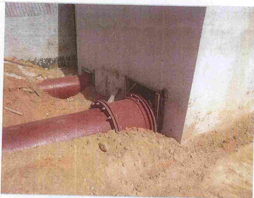
FOTO 17 – Chegada da tubulação DN 600 mm na CF1.
