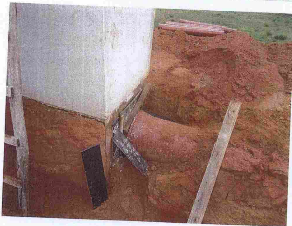
FOTO 6 - Vista da saída na CF2 da tubulação de interligação do sistema Ø400 mm..
