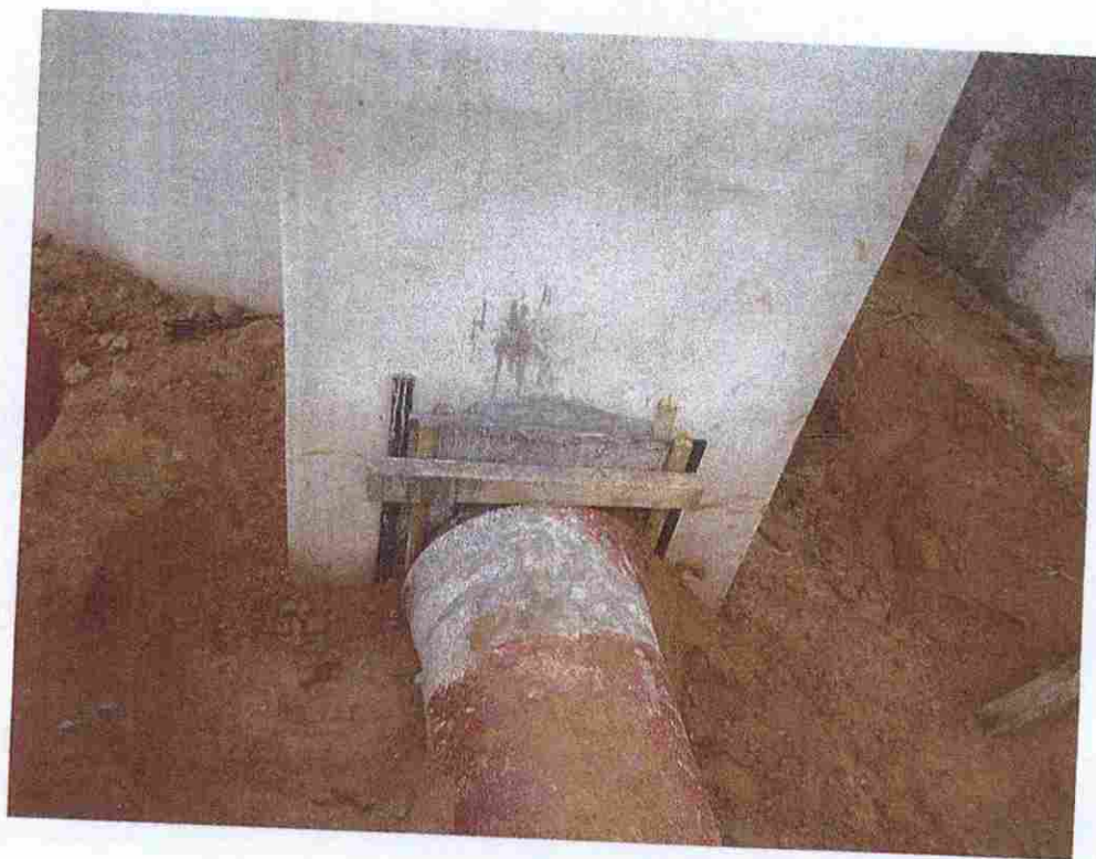
FOTO 5 - Vista da entrada na CF1 da tubulação de interligação do sistema Ø600 mm.
