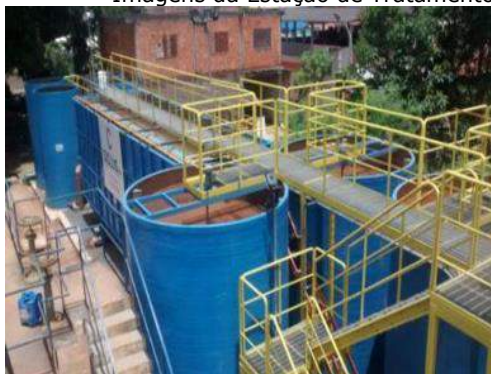
Imagens da Estação de Tratamento de Água Modular de Cachoeira Escura
