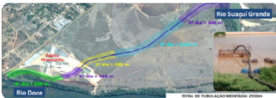
Figura 79: Adutora do Rio Suaçuí Grande para a ETA Recanto dos Sonhos, com capacidade de transporte de até 32 L/s. Em detalhe, balsa de captação no Rio Suaçuí Grande.
