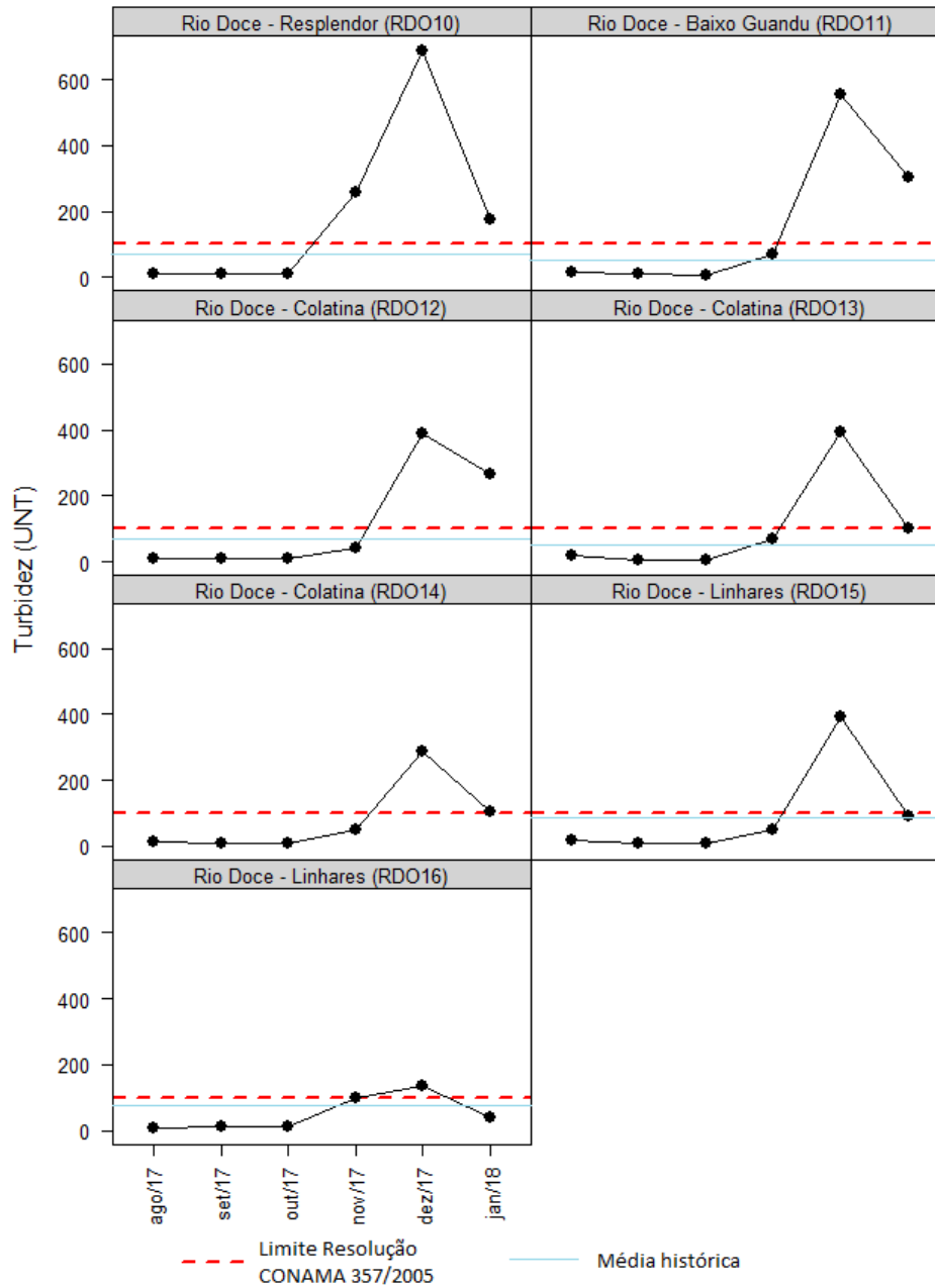
Figura 6-4b - Resultados de turbidez de sete pontos no rio Doce, de agosto/2017 a janeiro/2018.
