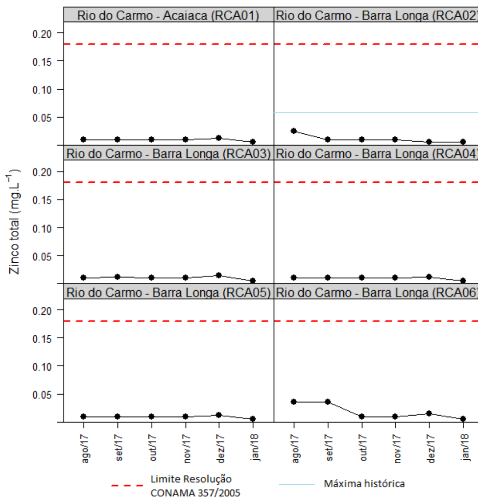
Figura 6-45 - Resultados de zinco total de seis pontos no rio do Carmo, de agosto/2017 a janeiro/2018.
