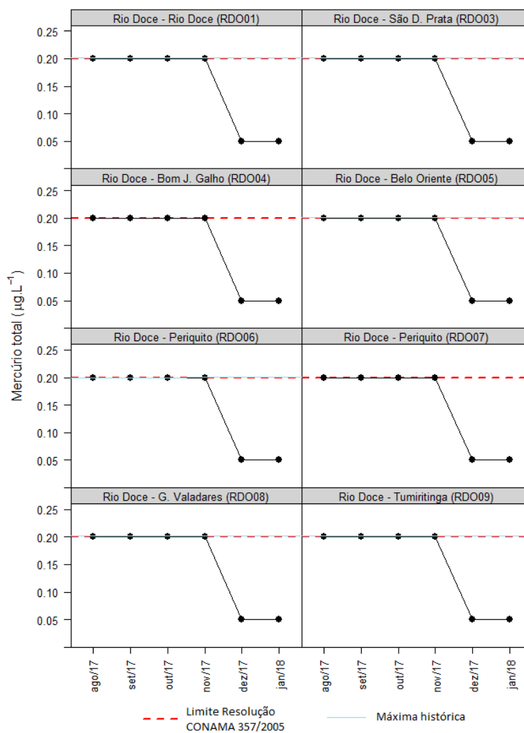
Figura 6-43b - Resultados de mercúrio total de sete pontos no rio Doce, de agosto/2017 a janeiro/2018.
