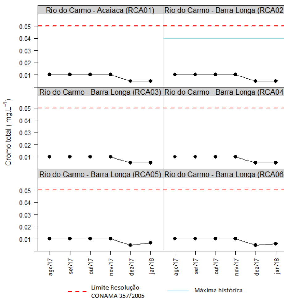
Figura 6-30 - Resultados de cromo total de seis pontos no rio do Carmo, de agosto/2017 a janeiro/2018.
