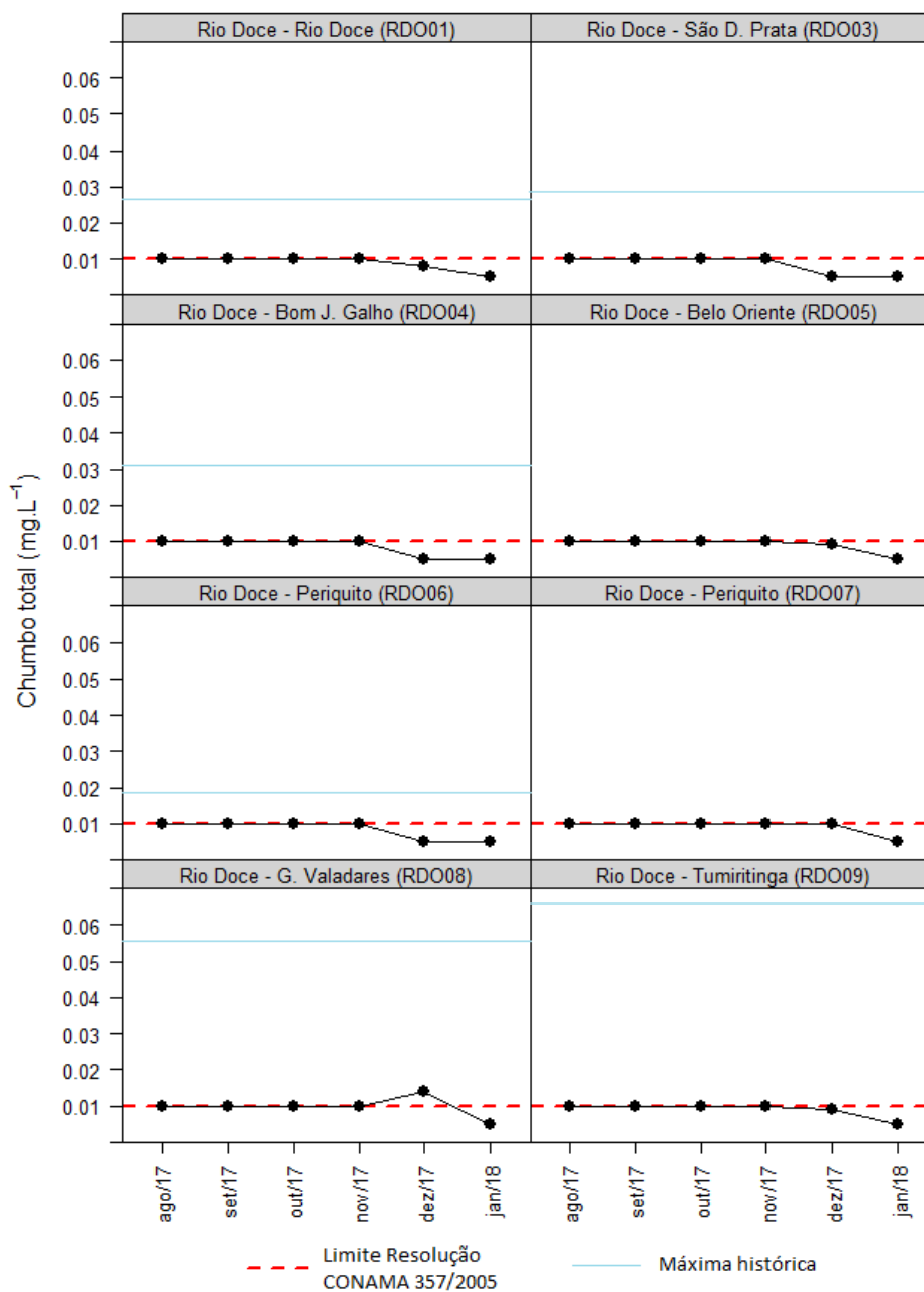
Figura 6-34a - Resultados de chumbo total de oito pontos no rio Doce, de agosto/2017 a janeiro/2018.
