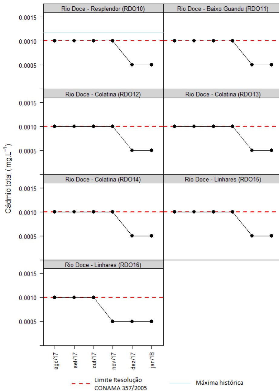
Figura 6-37b - Resultados de cádmio total de sete pontos no rio Doce, de agosto/2017 a janeiro/2018.
