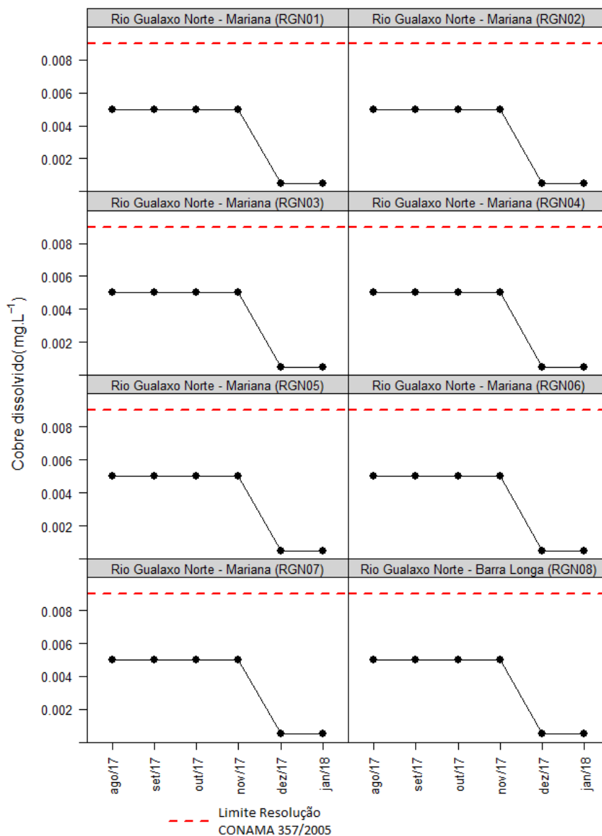
Figura 6-26 - Resultados de cobre dissolvido de oito pontos no rio Gualaxo do Norte, de agosto/2017 a janeiro/2018.
