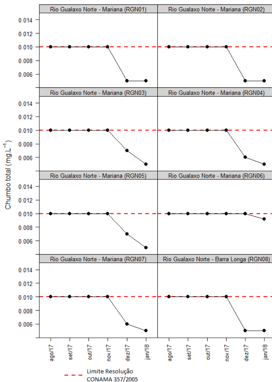
Figura 6-32 - Resultados de chumbo total de oito pontos no rio Gualaxo do Norte, de agosto/2017 a janeiro/2018.
