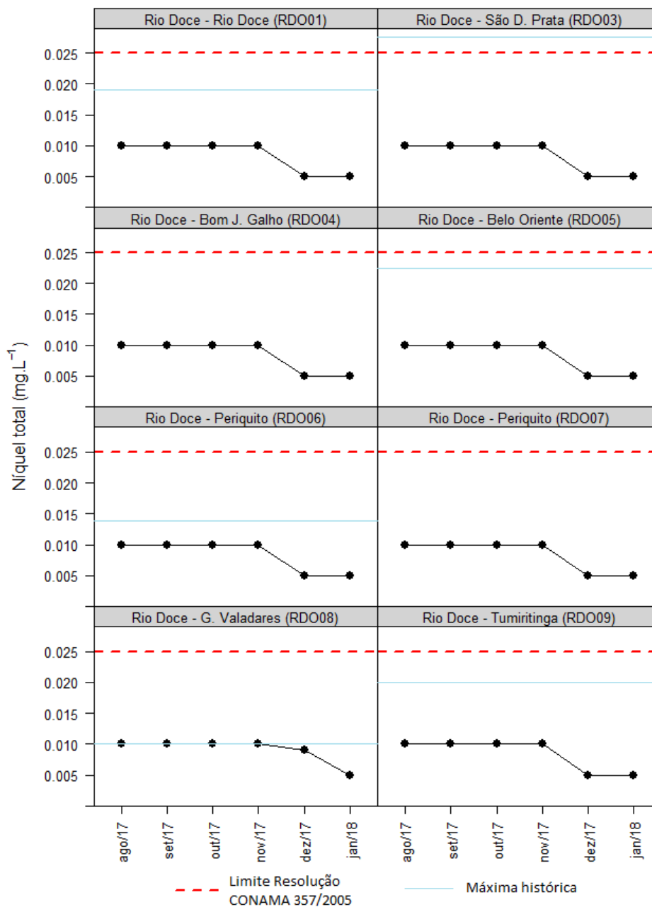
Figura 6-40a - Resultados de níquel total de seis pontos no rio do Carmo, de agosto/2017 a janeiro/2018.
