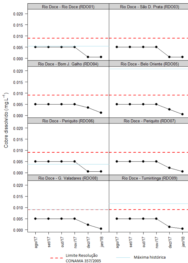
Figura 6-28a - Resultados de cobre dissolvido de oito pontos no rio Doce, de agosto/2017 a janeiro/2018.
