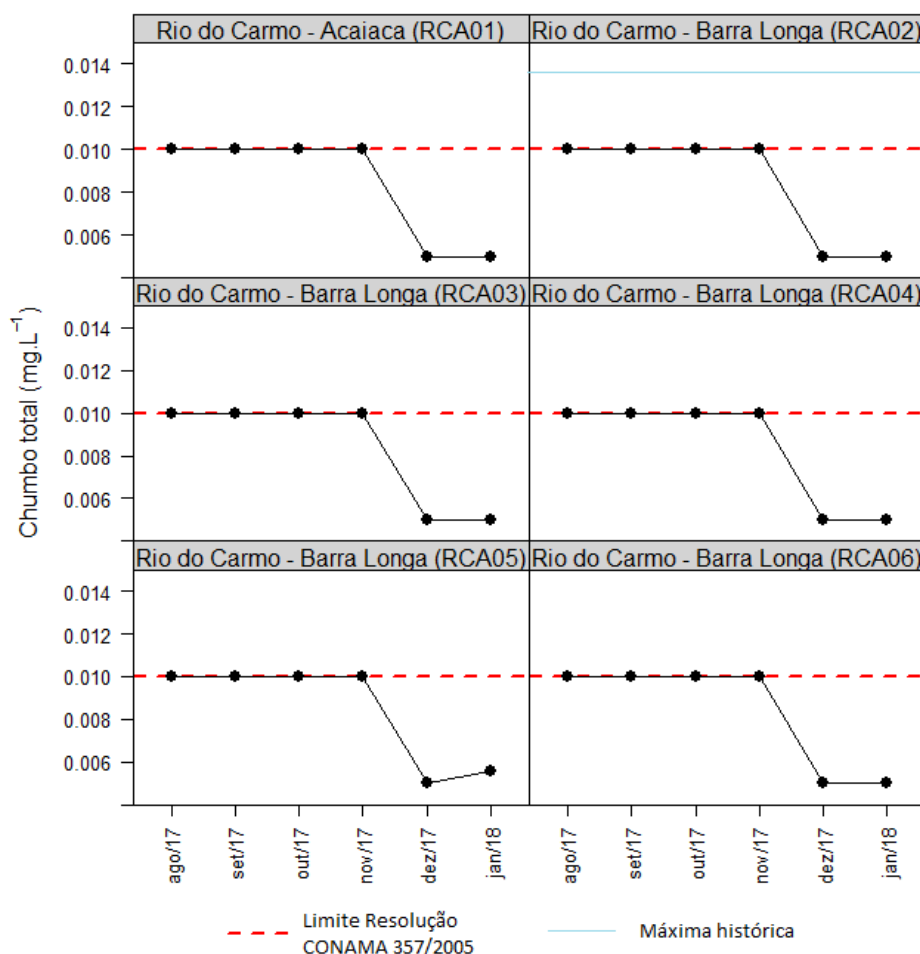
Figura 6-33 - Resultados de chumbo total de seis pontos no rio do Carmo, de agosto/2017 a janeiro/2018.
