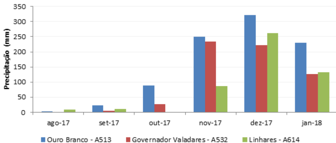
Figura 6-1 – Chuva acumulada mensal para três estações do INMET localizadas na bacia do rio Doce, de agosto de 2017 a janeiro de 2018.
