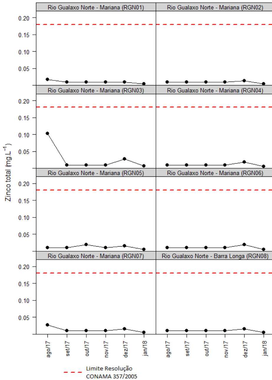
Figura 6-44 - Resultados de zinco total de oito pontos no rio Gualaxo do Norte, de agosto/2017 a janeiro/2018.
