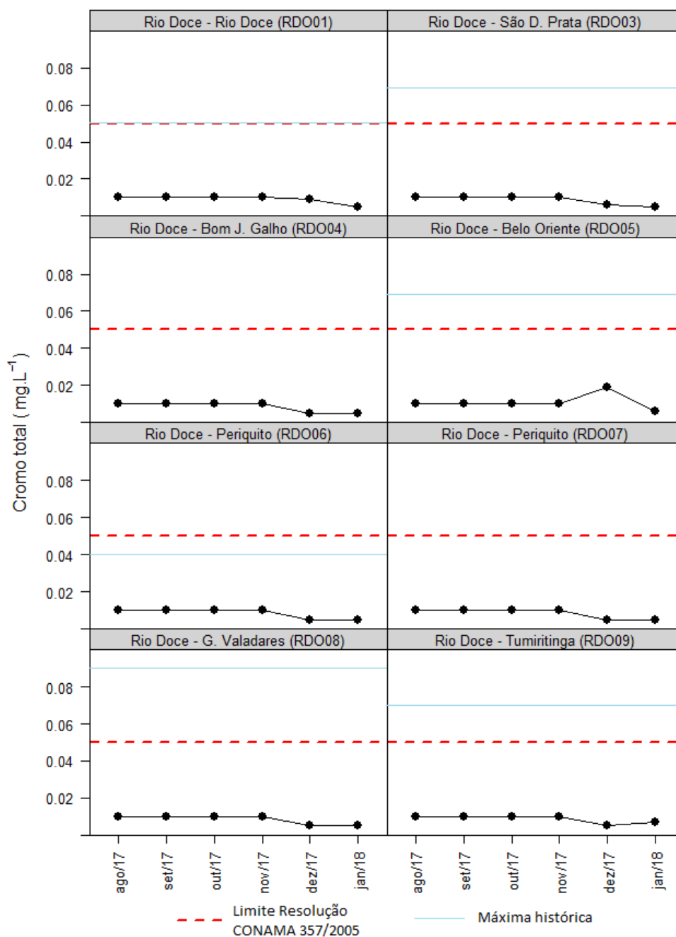
Figura 6-31a - Resultados de cromo total de oito pontos no rio Doce, de agosto/2017 a janeiro/2018.
