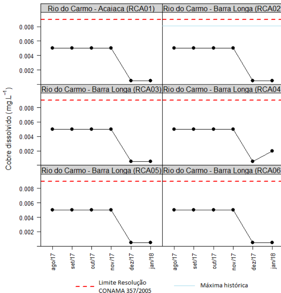
Figura 6-27 - Resultados de cobre dissolvido de seis pontos no rio do Carmo, de agosto/2017 a janeiro/2018.
