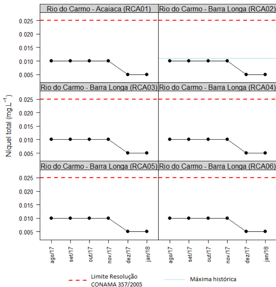
Figura 6-39 - Resultados de níquel total de seis pontos no rio do Carmo, de agosto/2017 a janeiro/2018.
