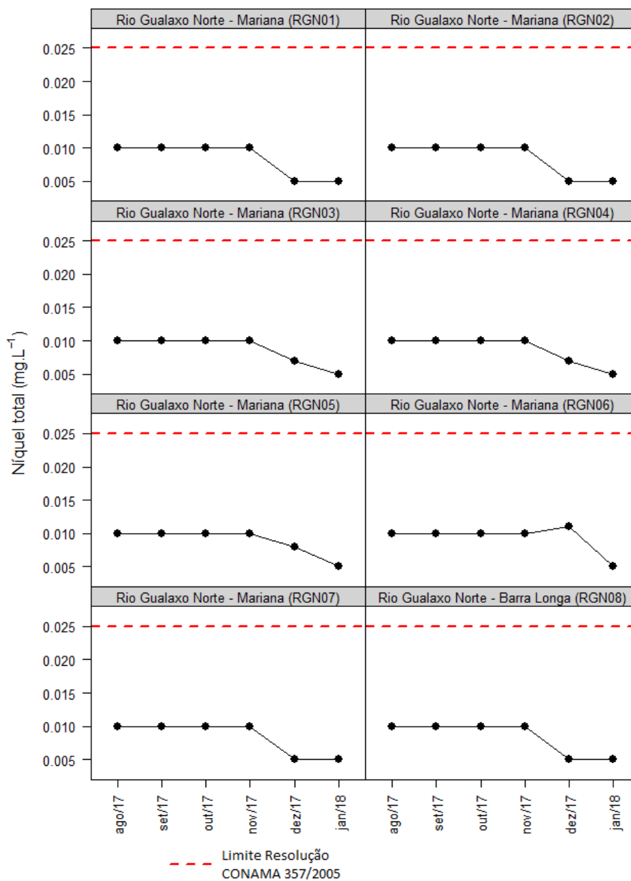
Figura 6-38 - Resultados de níquel total de oito pontos no rio Gualaxo do Norte, de agosto/2017 a janeiro/2018.
