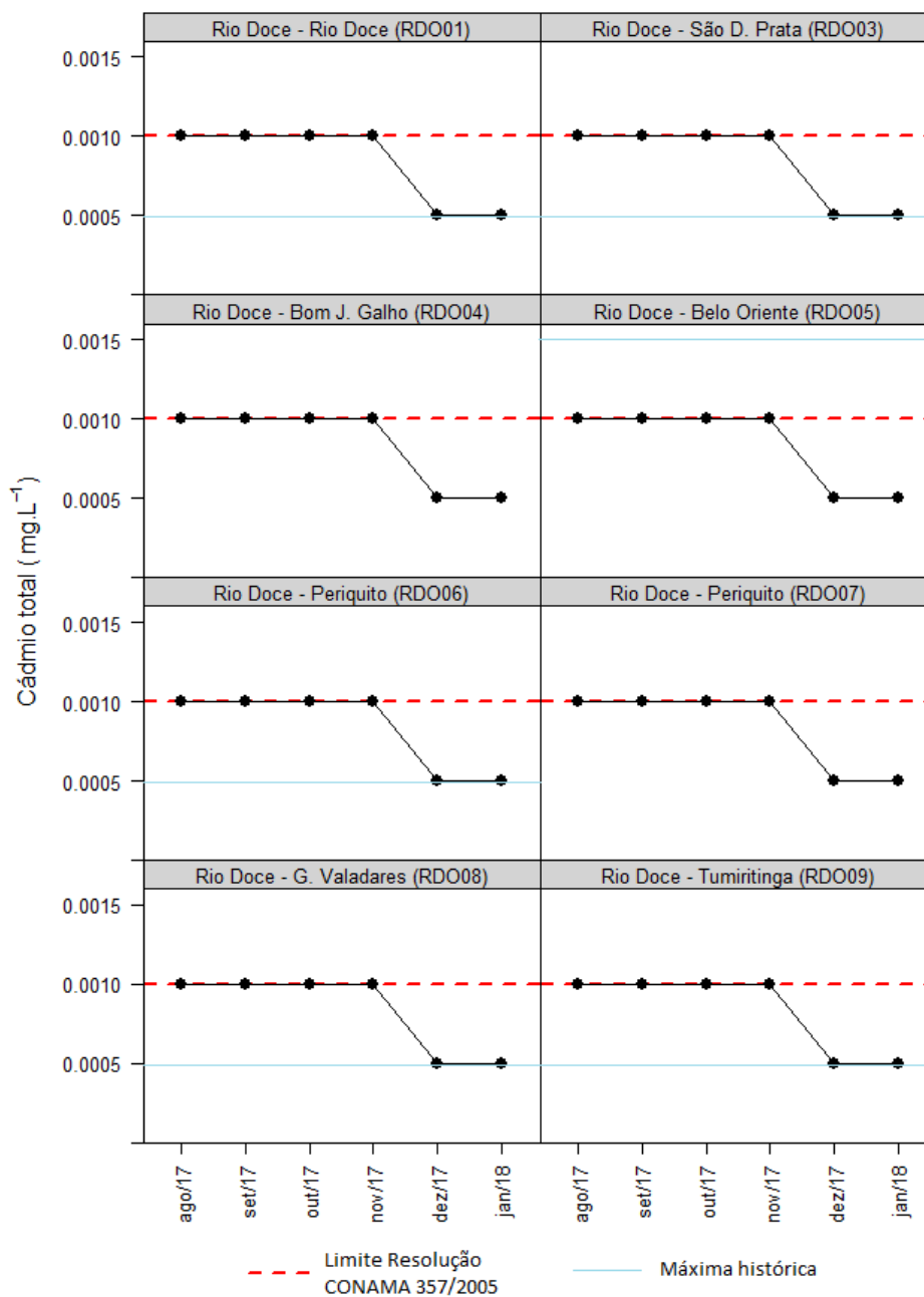
Figura 6-37a - Resultados de cádmio total de oito pontos no rio Doce, de agosto/2017 a janeiro/2018.
