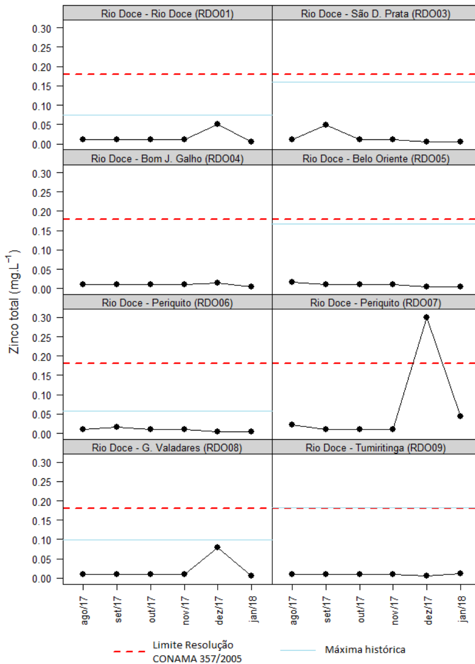
Figura 6-46a - Resultados de zinco total de oito pontos no rio Doce, de agosto/2017 a janeiro/2018.
