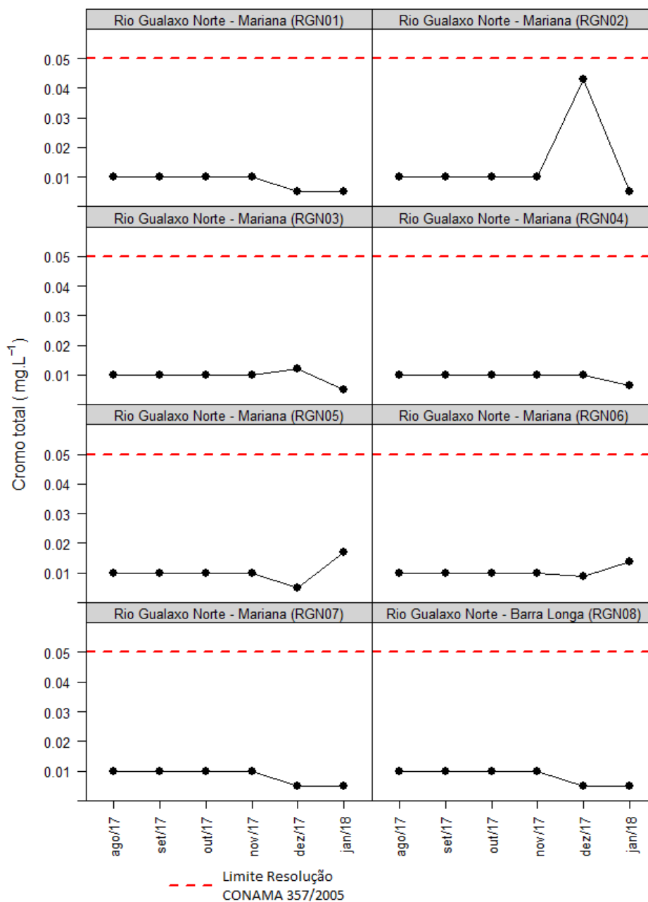
Figura 6-29 - Resultados de cromo total de oito pontos no rio Gualaxo do Norte, de agosto/2017 a janeiro/2018.
