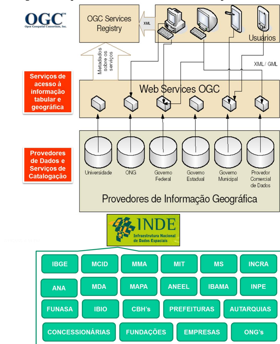
Figura 2: Esquema funcional da INDE incluindo provedores
