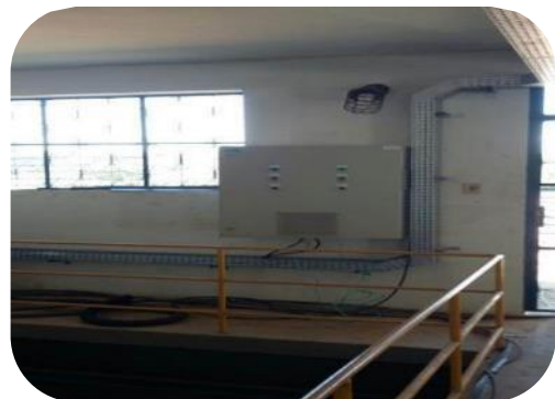
Figura 42: Novo painel (à esquerda) e eletrocalha (à direita) instalados na ETA 1 de Colatina.
