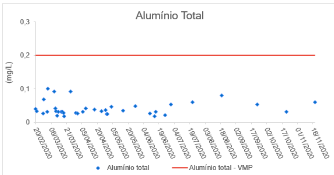
Figura 2: Monitoramento de Alumínio total (mg/L) na água tratada da ETA de Galileia
