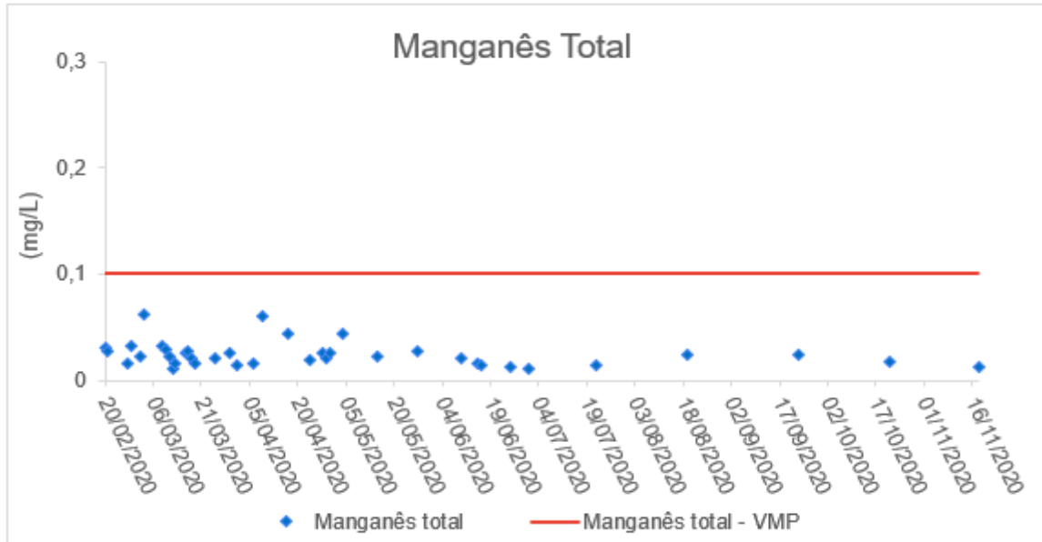
Figura 4: Monitoramento de Manganês total (mg/L) na água tratada da ETA de Galileia
