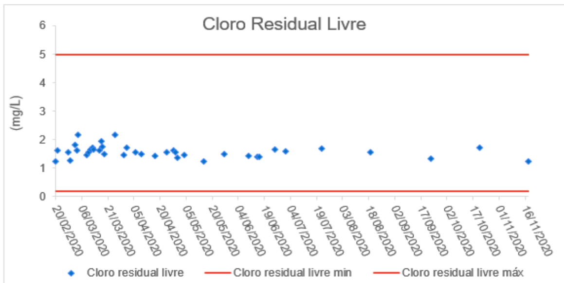
Figura 5: Monitoramento de Cloro residual livre (mg/L) na água tratada da ETA de Galileia
