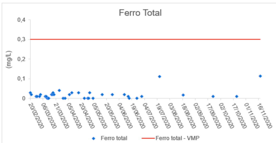
Figura 3: Monitoramento de Ferro total (mg/L) na água tratada da ETA de Galileia
