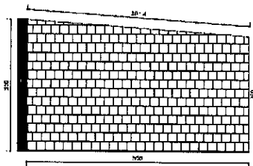
CORTE B-B - GARAGEM
