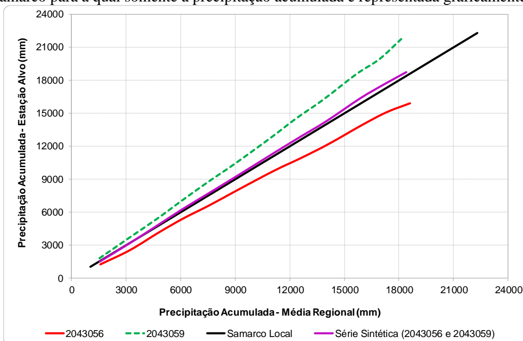
Figura 5: Curvas de Dupla Massa.
