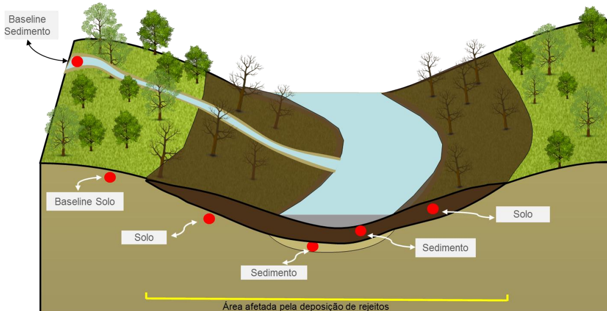
Figura 4: Desenho esquemático representando os tipos de materiais amostrados e analisados nos estudos geoquímicos.
