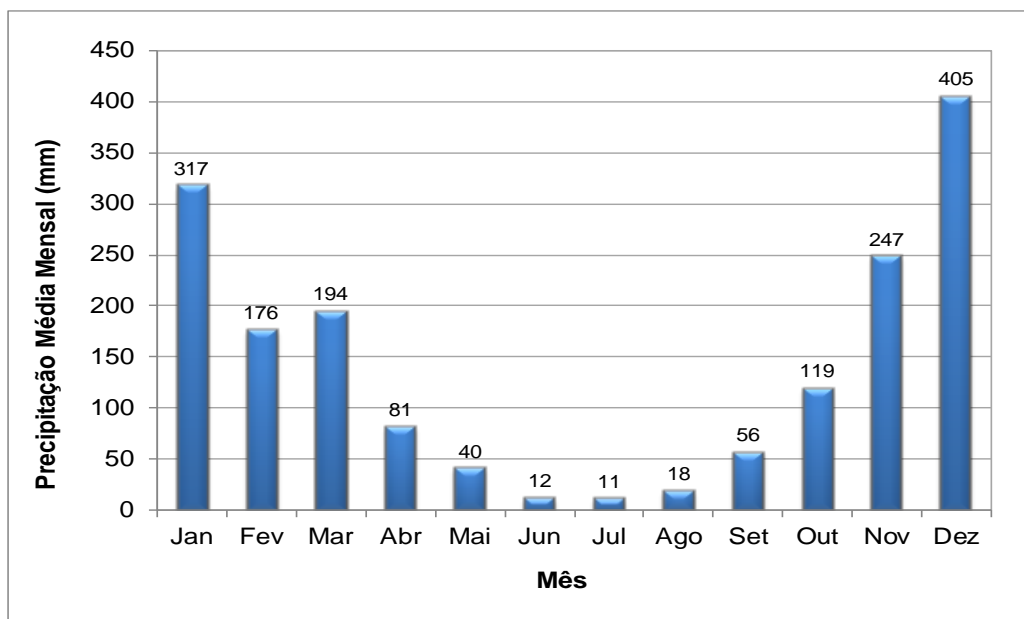
Figura 6: Variação Média Mensal da Precipitação da Série Sintética – Fazenda Água Limpa Jusante (Código ANA 2043056) e Colégio Caraça (Código ANA 2043059).
