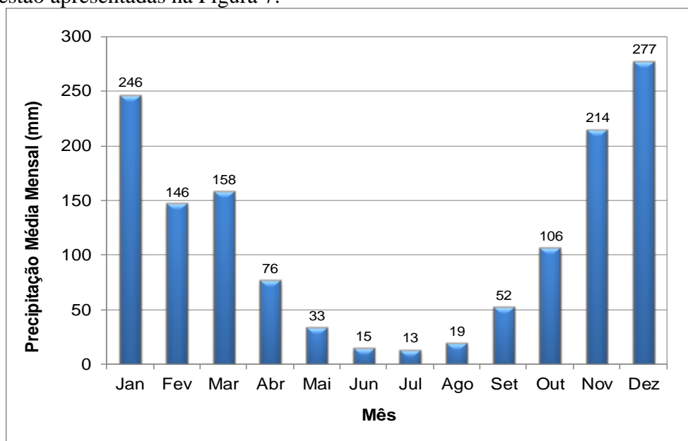
Figura 7: Variação Média Mensal da Precipitação da Série de Histórica – Fazenda Ocidente (código ANA 2043027)
