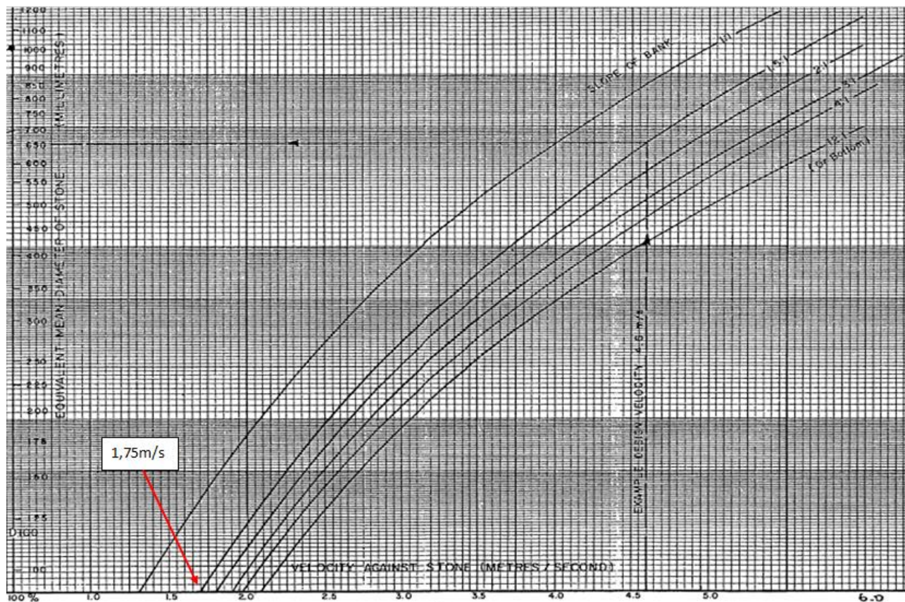
Figura 10: Velocidade do escoamento x D50 para diferentes declividades de talude
