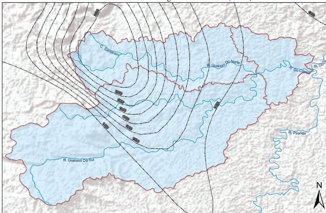
Figura 9: Isoietas anuais médias nas bacias dos rios Gualaxo do Norte e do Carmo.
