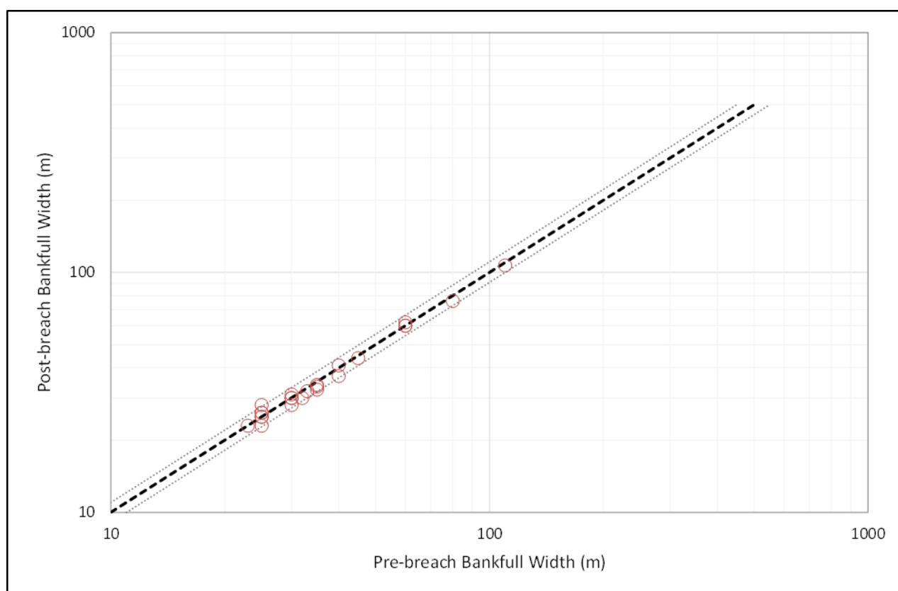
Figura 3: Comparação de larguras do leito menor pré e pós-rompimento; a linha representa uma comparação 1 a 1, com limites de \pm 10\% .
