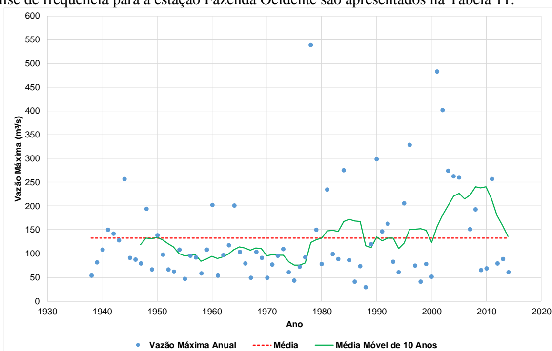
Figura 8: Vazões Máximas Anuais da Série Histórica – Fazenda Ocidente (Código ANA 56337000).
