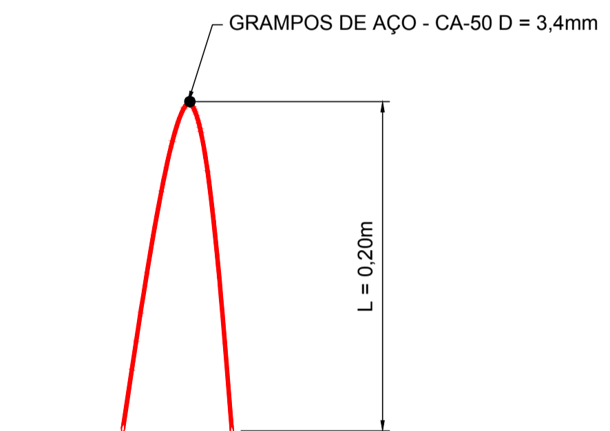
SEM ESCALA 5 DETALHE DO GRAMPO
