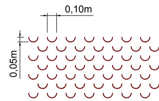
SEM ESCALA 1 DETALHE DO COVEAMENTO
