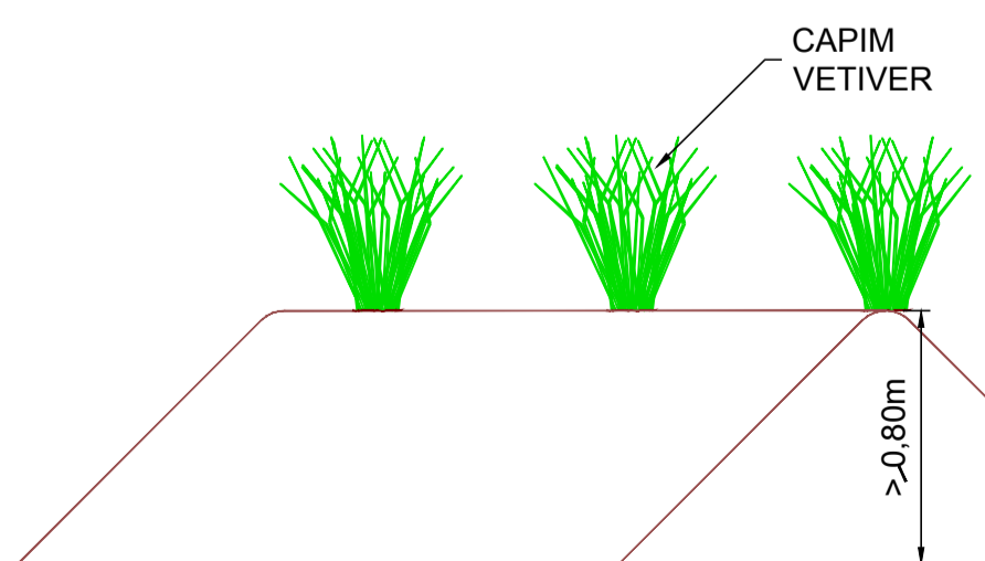
SEM ESCALA 6 DETALHES DO PLANTIO DAS MUDAS DE CAPIM VETIVER
