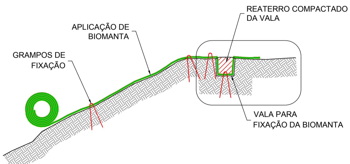
SEM ESCALA 3 DETALHES DO ANCORAMENTO DA BIOMANTA
