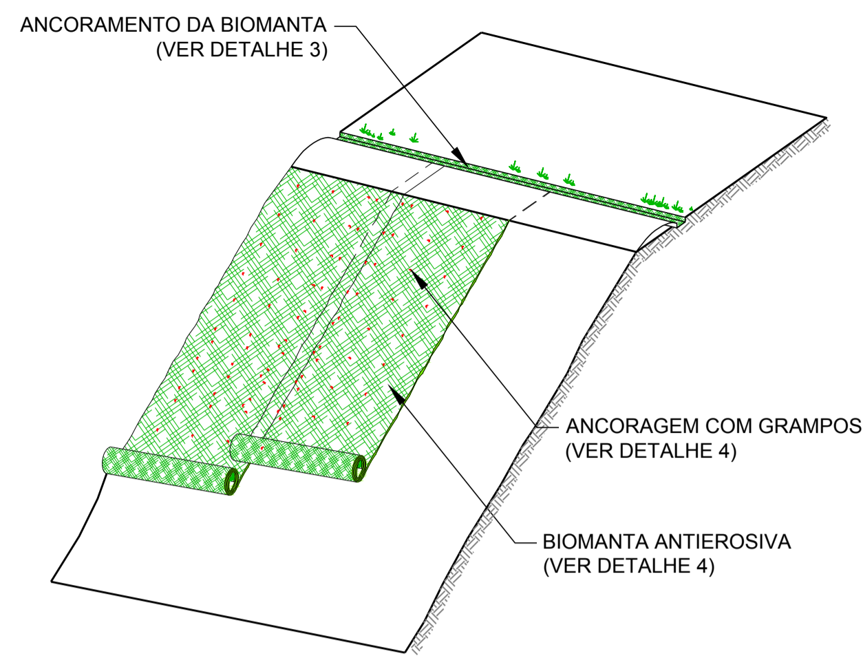
BIOMANTA SEM ESCALA
