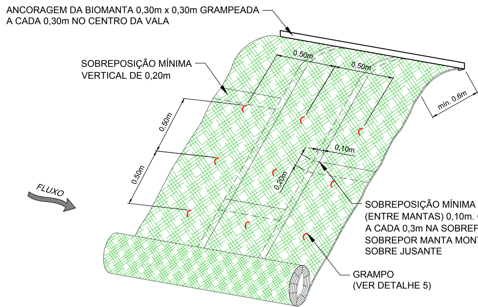
SEM ESCALA 4 DETALHE DA APLICAÇÃO DA BIOMANTA
