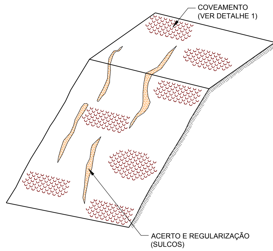
PREPARO DO SOLO SEM ESCALA
