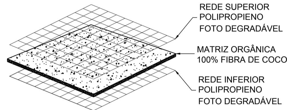
TIPOS DE BIOMANTA SEM ESCALA
