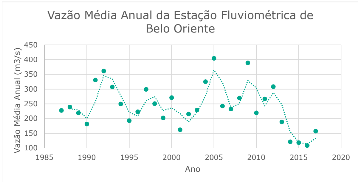
Figura 30: Vazão Média (m³/s) – Estação Belo Oriente
