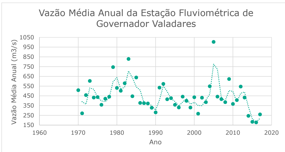
Figura 31: Vazão Média (m³/s) – Estação Governador Valadares
