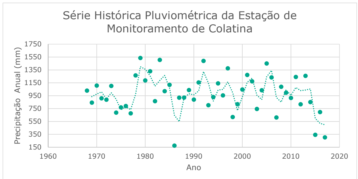
Figura 29: Precipitação Anual (mm) – Estação Colatina
