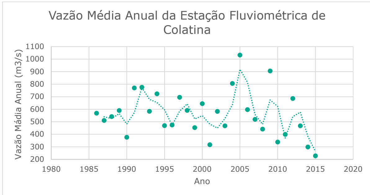
Figura 32: Vazão Média (m 3 /s) – Estação Colatina
