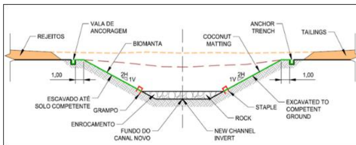
Figura 20: Exemplo de seção típica para a recuperação dos tributários – Biomanta e Enrocamento (Opção 10). Fonte: Projeto Golder Associates.
