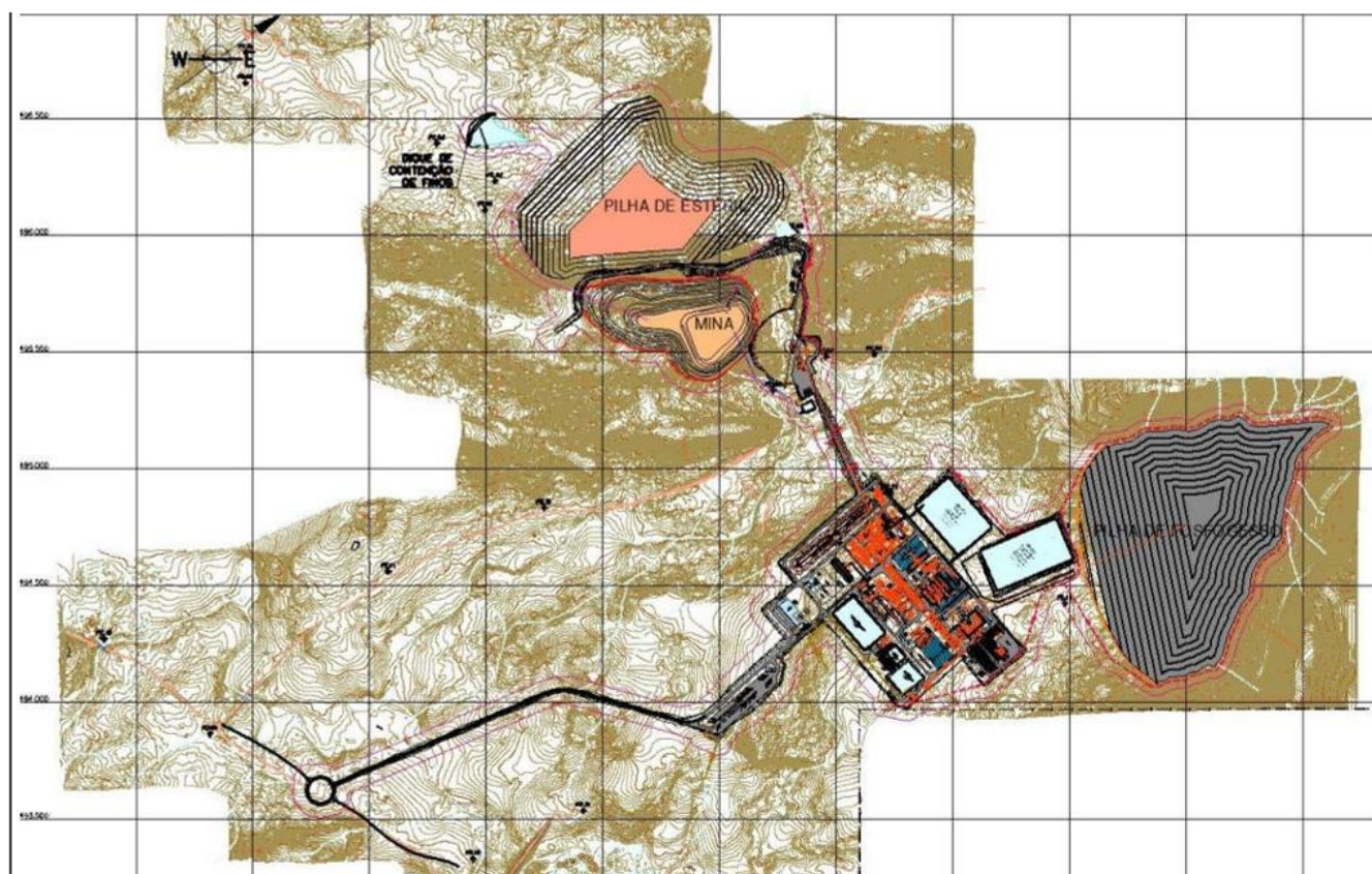
Figura 7 – Arranjo Geral do Projeto Santa Quitéria.
