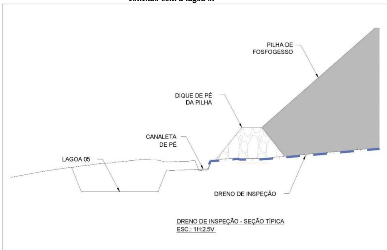
Figura 9 – Seção Transversal típica do pé da pilha de Fosfogesso e Cal mostrando sua conexão com a lagoa 5.
