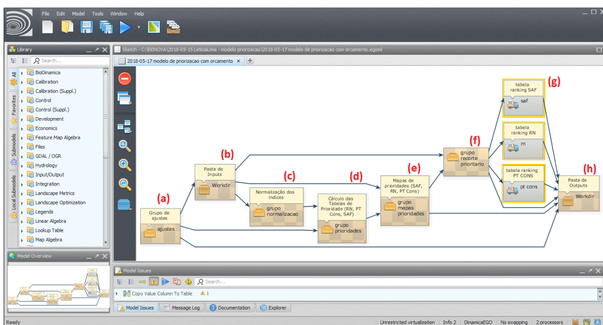
Figura 70. Visão Geral do modelo computacional de priorização implementado na plataforma de modelagem Dinamica EGO.
