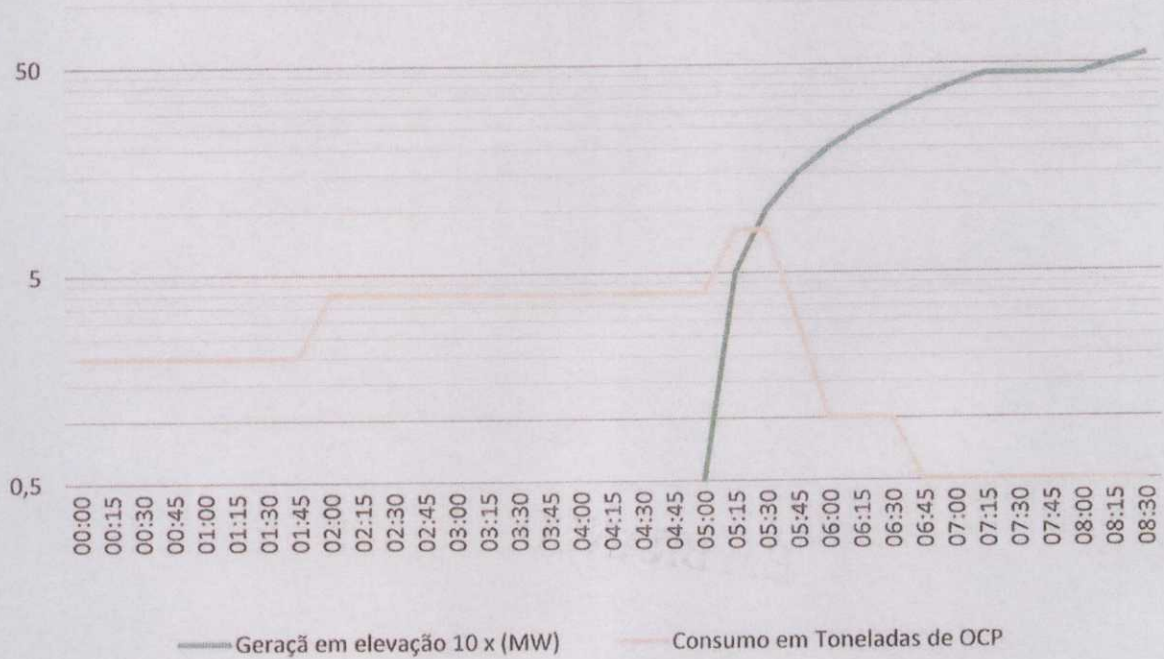
Gráfico 1 - Acendimento típico da Unidade 1
