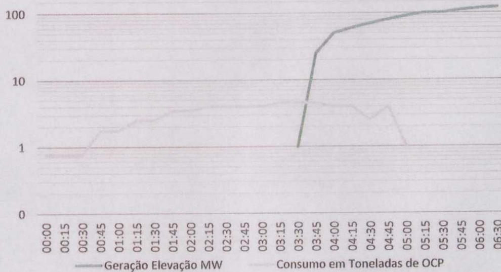
Gráfico 4 - Gráfico típico de acendimento Unidade 4
