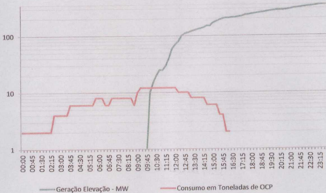
Gráfico 5 - Curva típica de acendimento da Unidade 5
