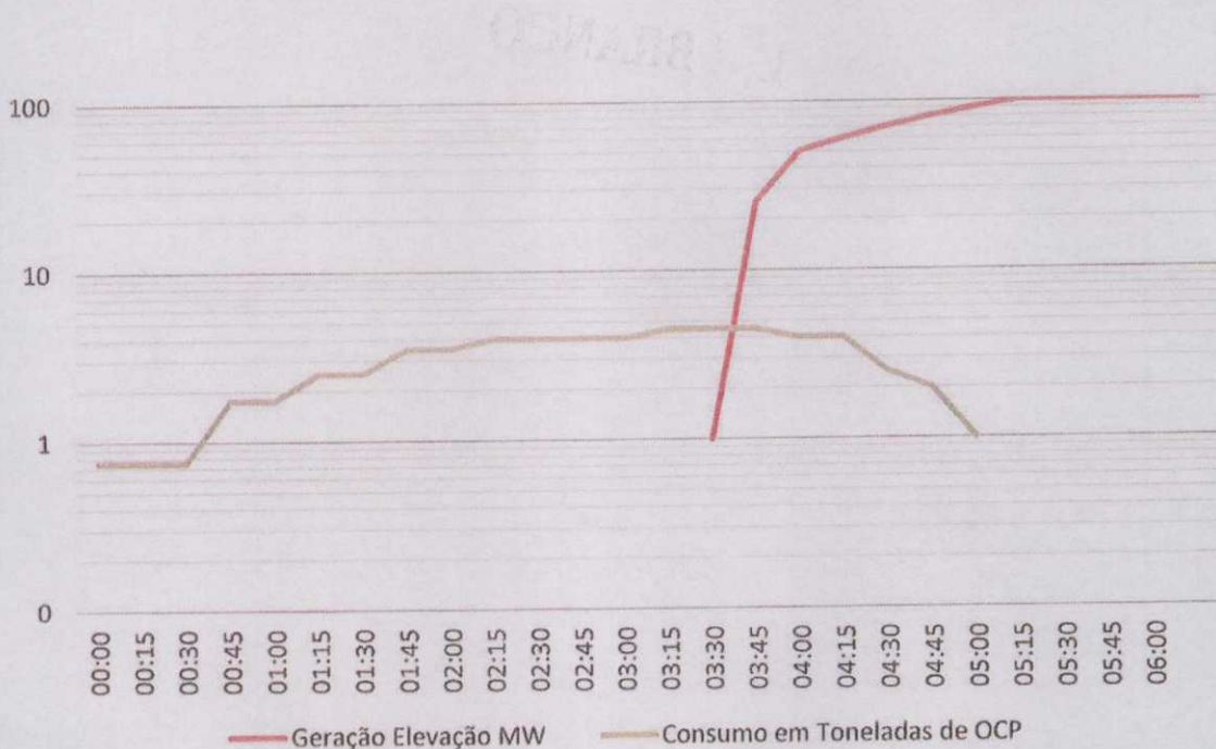
Gráfico 3 - Gráfico típico de acendimento da Unidade 3
