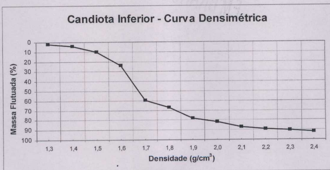
Figura 2: Curva de lavabilidade do Banco Inferior.
