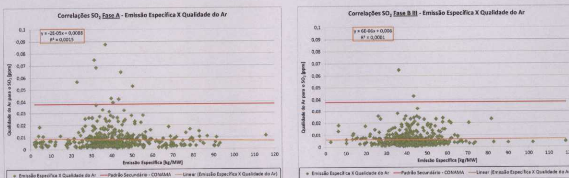
Figura 10. Correlações de Emissão Específica e Qualidade do Ar para a Fase A e Unidade III da Fase B.
