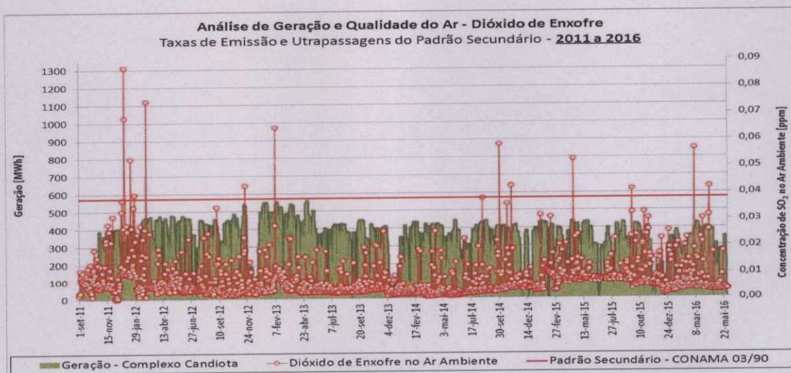
Figura 18. Geração nas Fases A, B e C e Qualidade do Ar para ao \text{SO}_2 no 6º Período avaliado.
