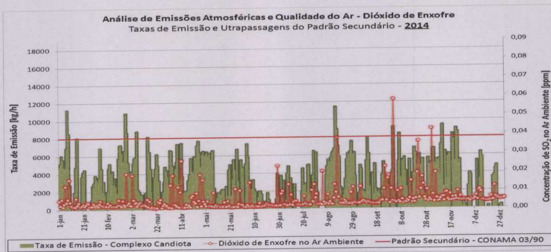
Figura 15. Taxa de emissão das Fases A, B e C e Qualidade do Ar para ao \text{SO}_2 no 3º Período avaliado.
