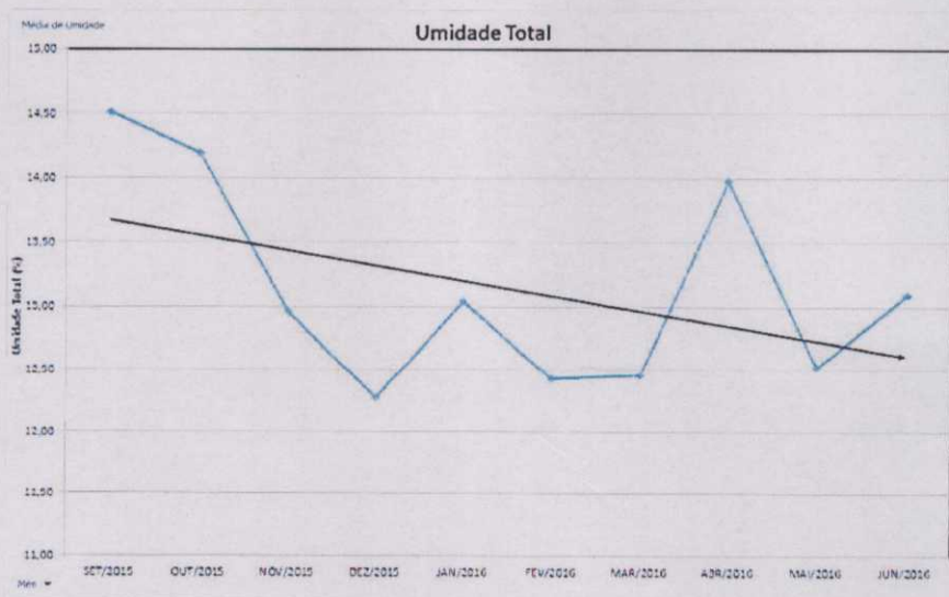
Figura 1 - Gráfico da Umidade Total
