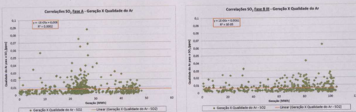
Figura 4. Correlações de Geração e Qualidade do Ar para a Fase A e Unidade III da Fase B.
