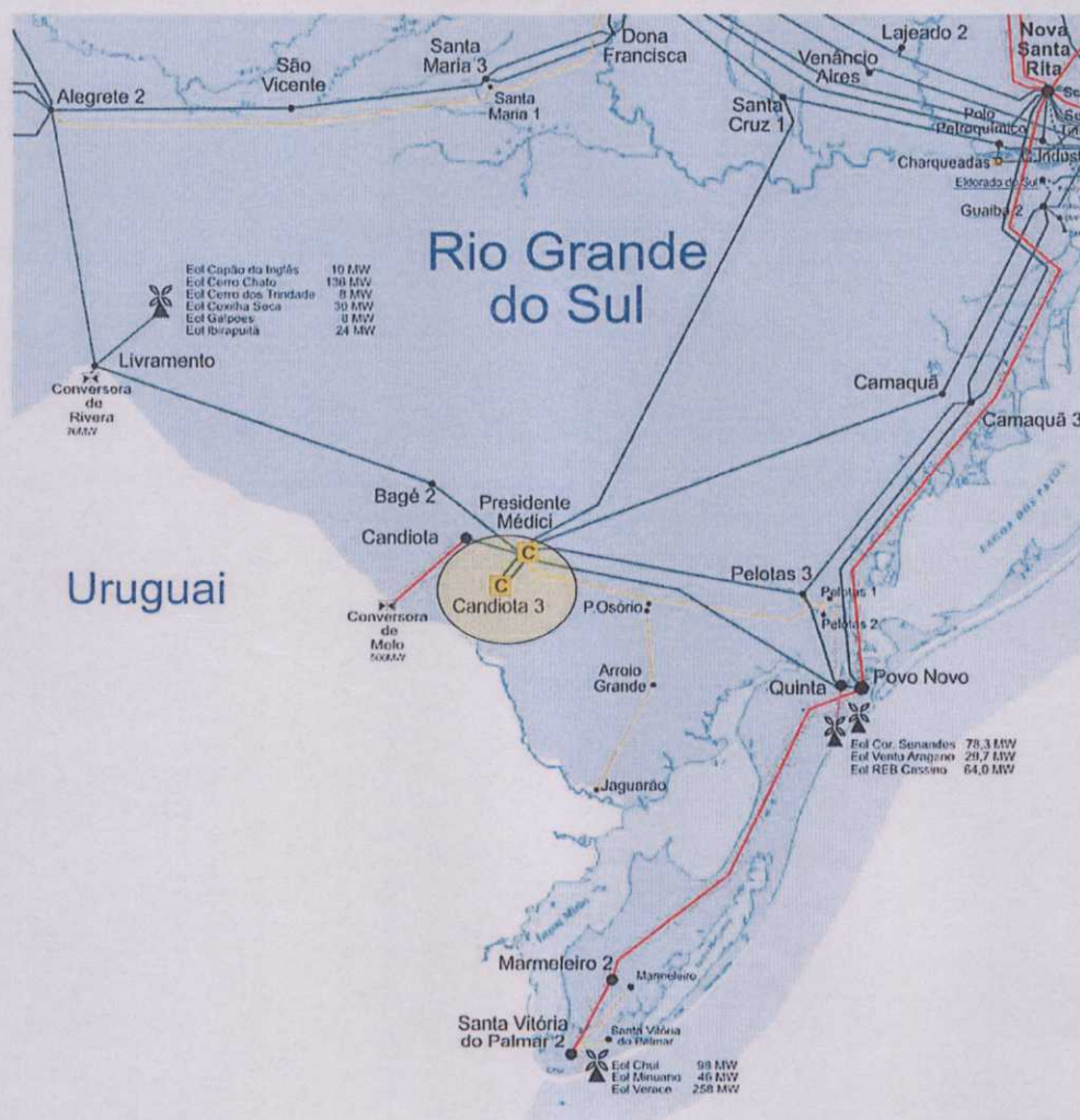
Figura 1-1: Conexão da UTE Candiota III ao SIN – diagrama geoeletrico
