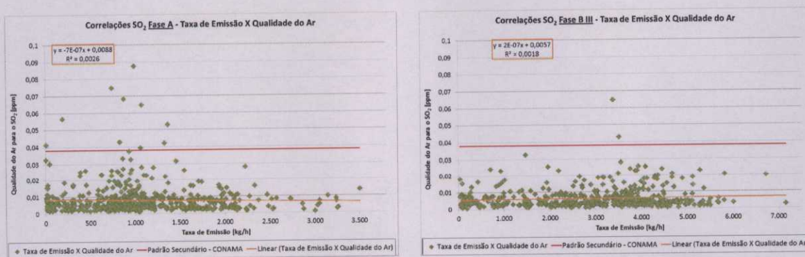
Figura 7. Correlações entre Taxa de Emissão e Qualidade do Ar para a Fase A e a Unidade III da Fase B.
