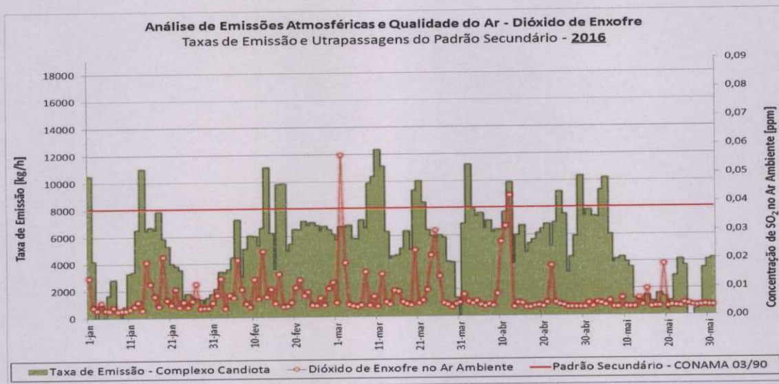
Figura 17. Taxa de emissão das Fases A, B e C e Qualidade do Ar para ao \text{SO}_2 no 5º Período avaliado.
