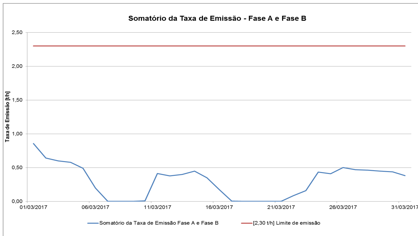
Figura 10. Taxa de emissão de Material Particulado das Fases A e B.
