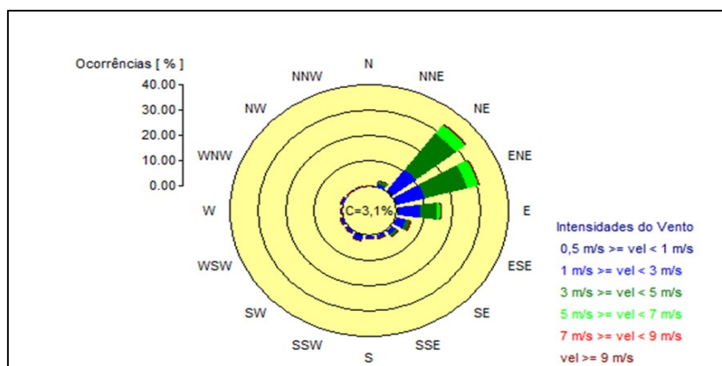
Figura 20 – Rosa dos Ventos – Estação Aceguá.
