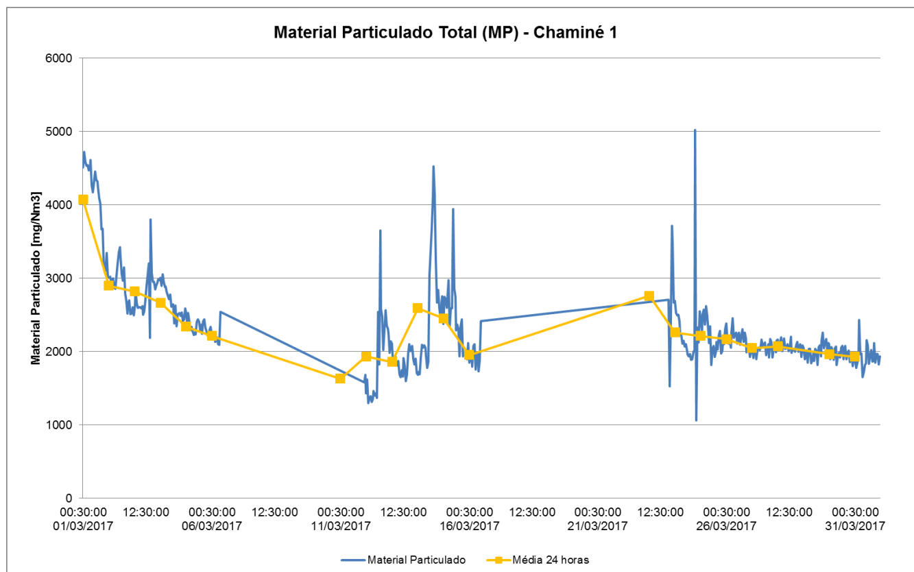
Figura 5. Material Particulado Total [mg/Nm 3 ] – Chaminé 1
