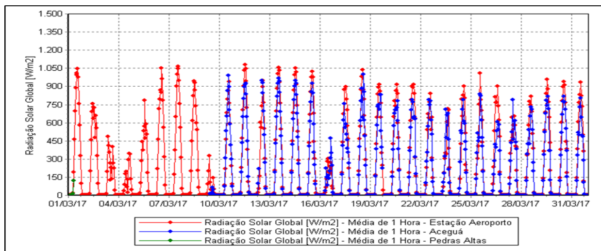
Figura 24 – Evolução das Medições de Radiação Solar.
