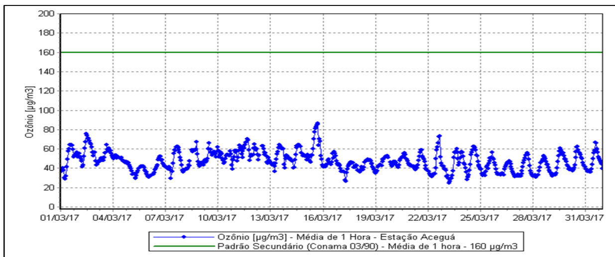
Figura 17 – Evolução das Concentrações de Ozônio – Estação Aceguá.
