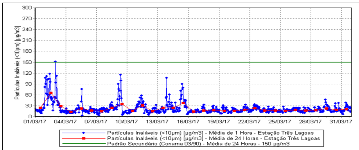
Figura 4 – Evolução da Concentração de Partículas Inaláveis - Estação Três Lagoas.
