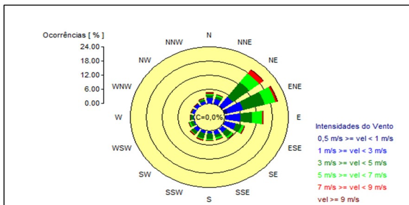
Figura 18 – Rosa dos Ventos – Estação Aeroporto.
