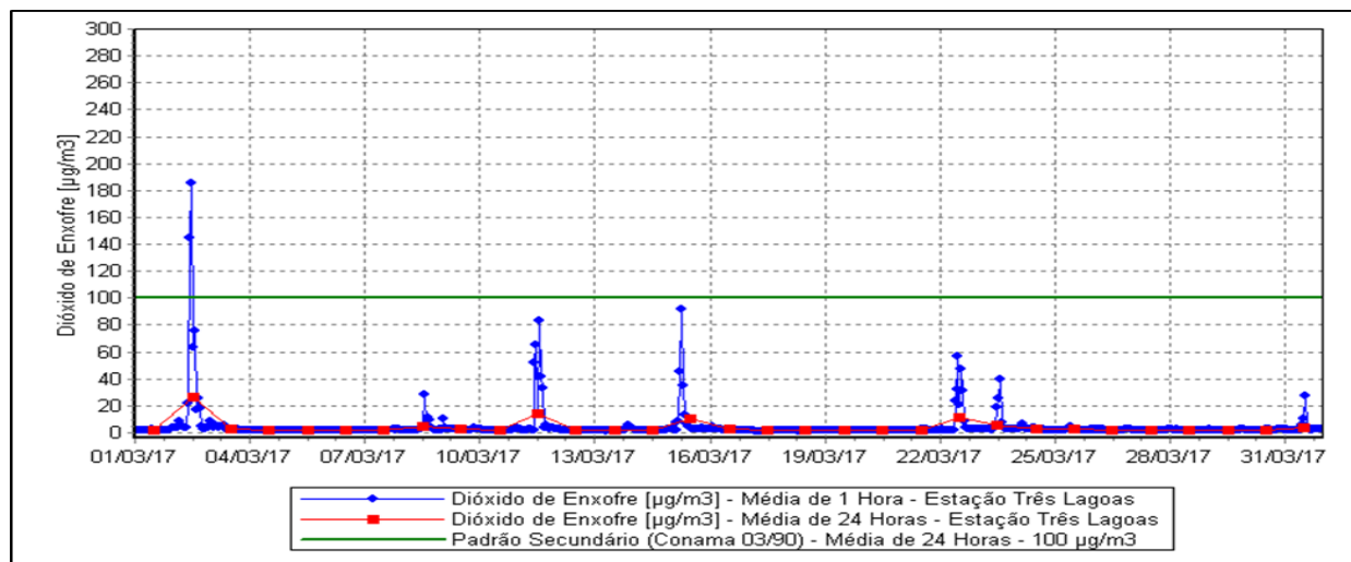
Figura 9 – Evolução das Concentrações de Dióxido de Enxofre – Estação Três Lagoas.
