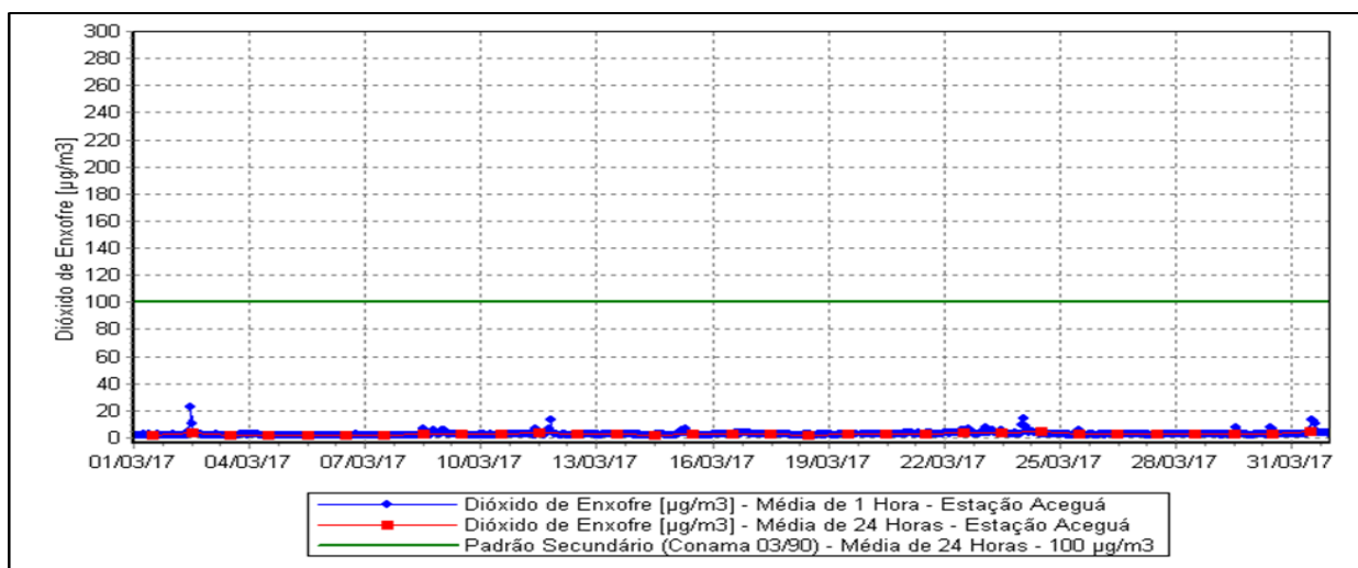
Figura 11 – Evolução das Concentrações de Dióxido de Enxofre – Estação Aceguá.
