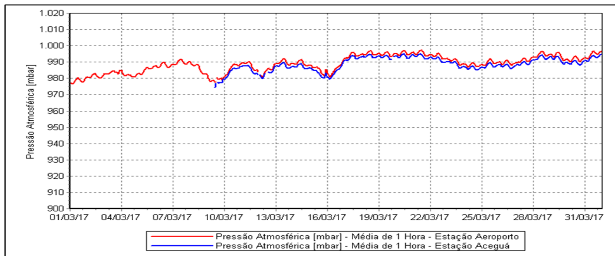
Figura 23 – Evolução das Medições de Pressão Atmosféricas.
