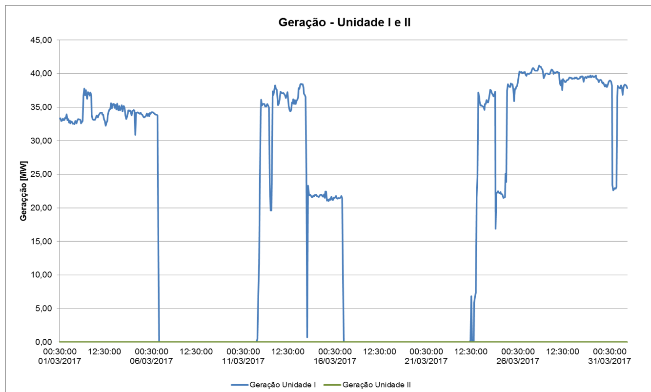
Figura 1. Geração de Energia - Fase A - Unidade I e II (Chaminé 1).
