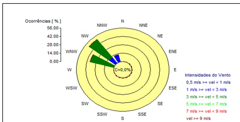
Figura 19 – Rosa dos Ventos – Estação Pedras Altas.
