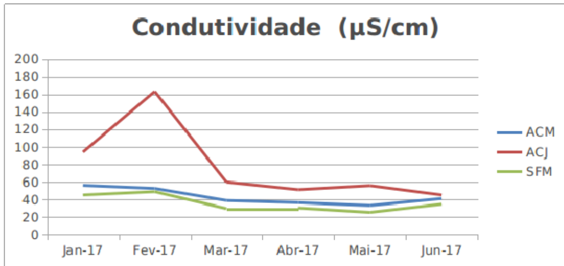
Gráfico 3 - Medições de Condutividade ( \mu\text{S}/\text{cm} ) para o período avaliado. Fonte: Ecosis, 2017.
