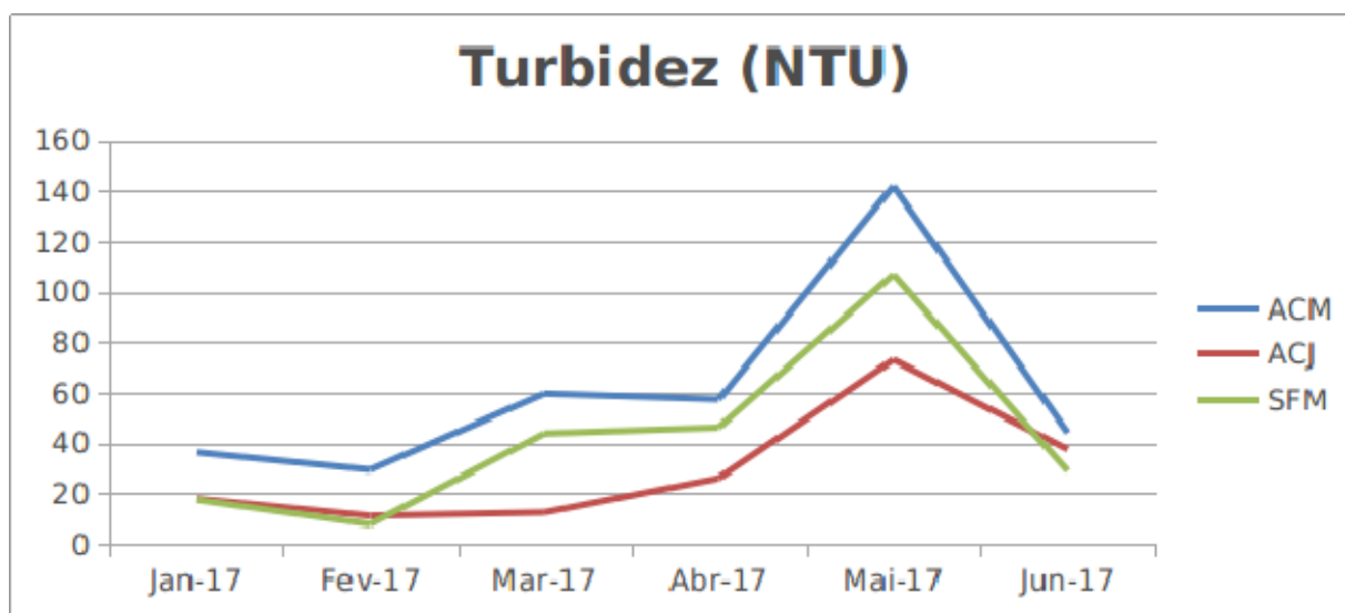
Gráfico 4 - Medições de Turbidez (NTU) para o período avaliado. Fonte: Ecosis, 2017.
