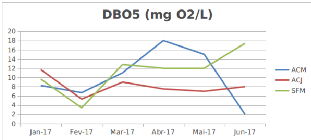
Gráfico 5 - Medições de DBO (mg O2/L) para o período avaliado. Fonte: Ecosis, 2017.
