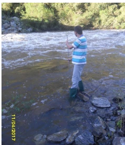
Figura 14 - Coleta de amostra para análise de sólidos em suspensão com o amostrador DH-48. Fonte: Ecosystems, 2017.
