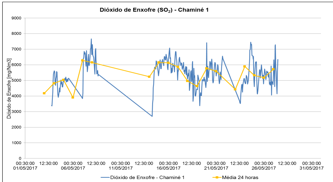
Figura 3. Dióxido de Enxofre [mg/Nm 3 ] – Chaminé 1
