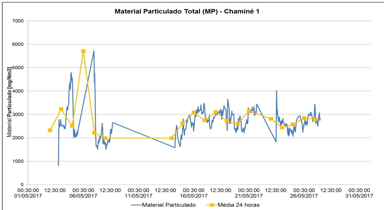
Figura 5. Material Particulado Total [mg/Nm 3 ] – Chaminé 1
