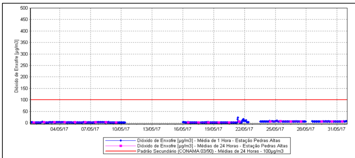
Figura 10 – Evolução das Concentrações de Dióxido de Enxofre – Estação Pedras Altas.
