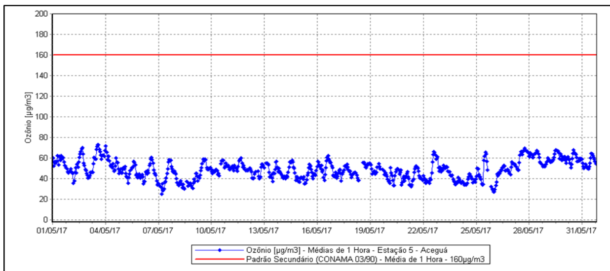
Figura 17 – Evolução das Concentrações de Ozônio – Estação Aceguá.
