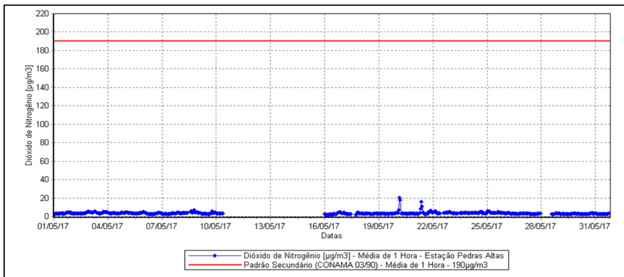
Figura 15 – Evolução das Concentrações de Dióxido de Nitrogênio – Estação Pedras Altas.
