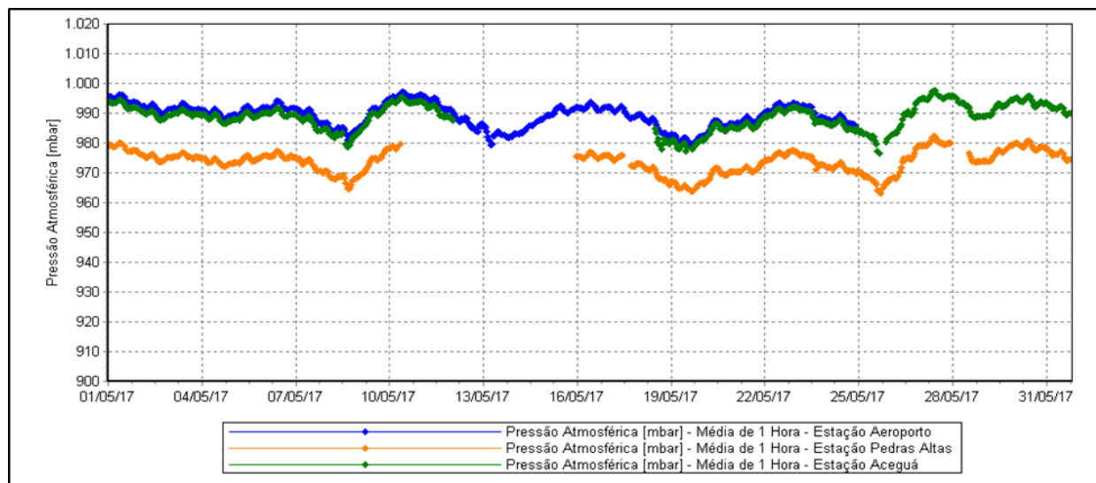
Figura 23 – Evolução das Medições de Pressão Atmosféricas.
