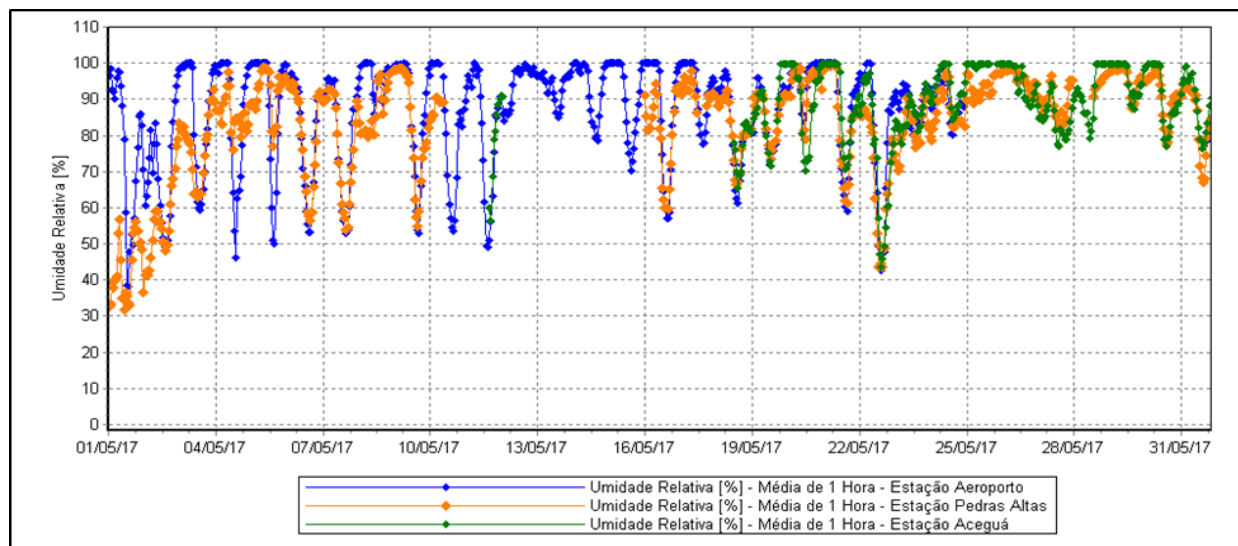
Figura 22 – Evolução das Medições de Umidade Relativa.
