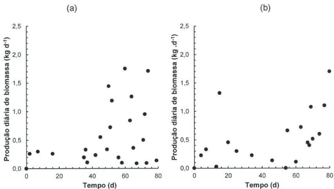
Figura 74: Produção diária de biomassa de Spirulina sp. LEB 18 no cultivo com injeção de gás de combustão (a) e no cultivo controle (b)
