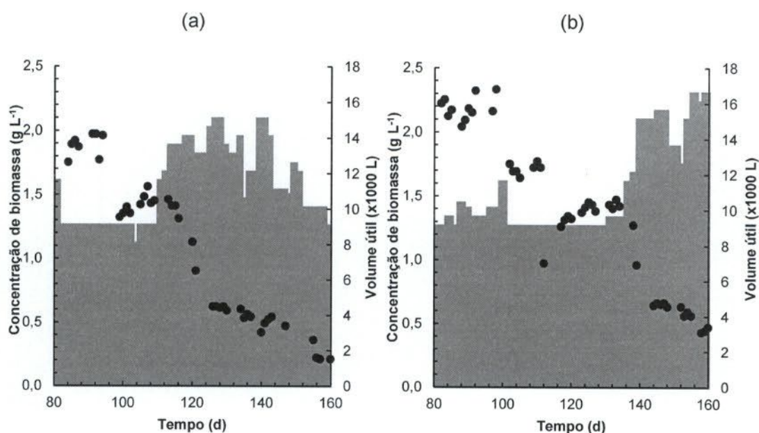
Figura 76: Concentração de biomassa de Spirulina sp. LEB 18 (●) e volume útil dos biorreatores (colunas cinzas) dos cultivos com gás de combustão (a) e controle (b) entre o 80º e 160º d
