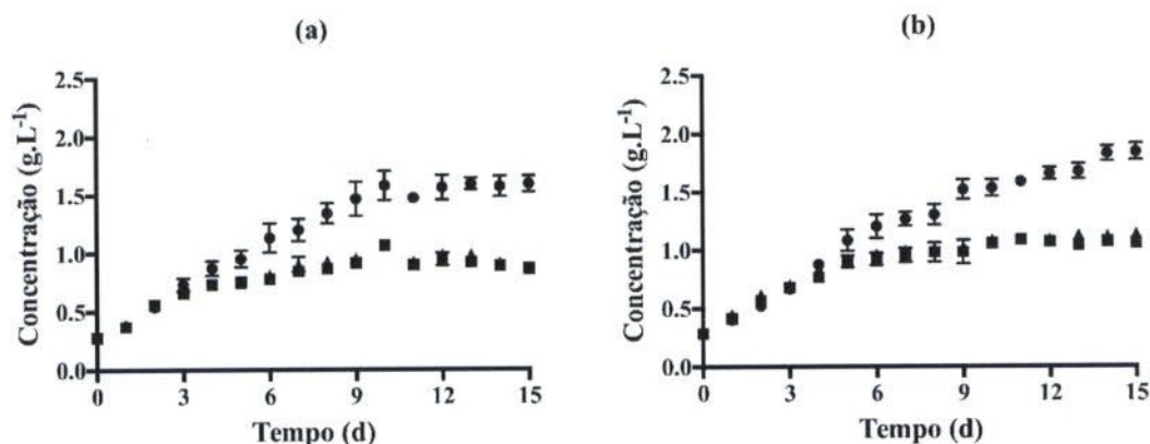
Figura 11: Perfil de crescimento de Chlorella minutissima com (a) 10% CO 2 e (b) 20% CO 2 , onde: (●) MBM Controle – 0,250 g.L -1 KNO 3 , (■) MBM – 0,125 g.L -1 KNO 3 e (▲) MBM – 0,125 g.L -1 KNO 3 + 19,16 mg.L -1 Xilose e 0,89 mg.L -1 Arabinose.
