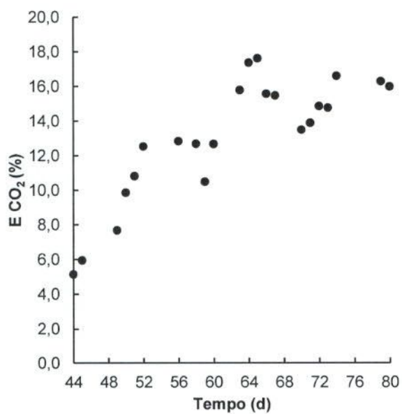
Figura 75: Eficiência de utilização de gás carbônico presente no gás de combustão
