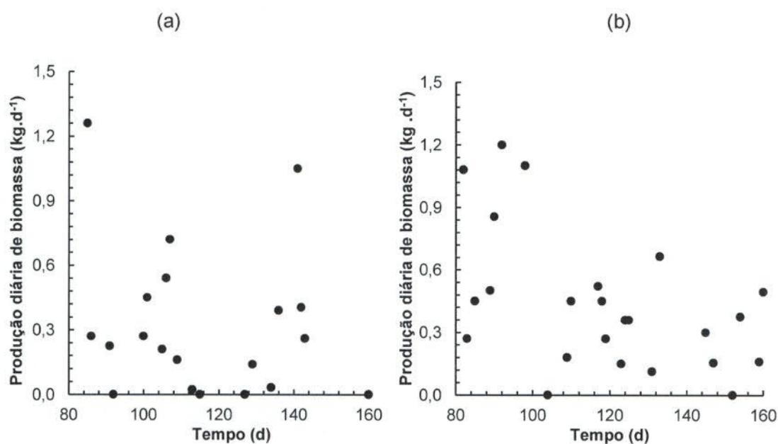
Figura 77: Produção de biomassa de Spirulina sp. LEB 18 no cultivo com gás de combustão (a) e no cultivo controle (b) entre o 80° e 160° d
