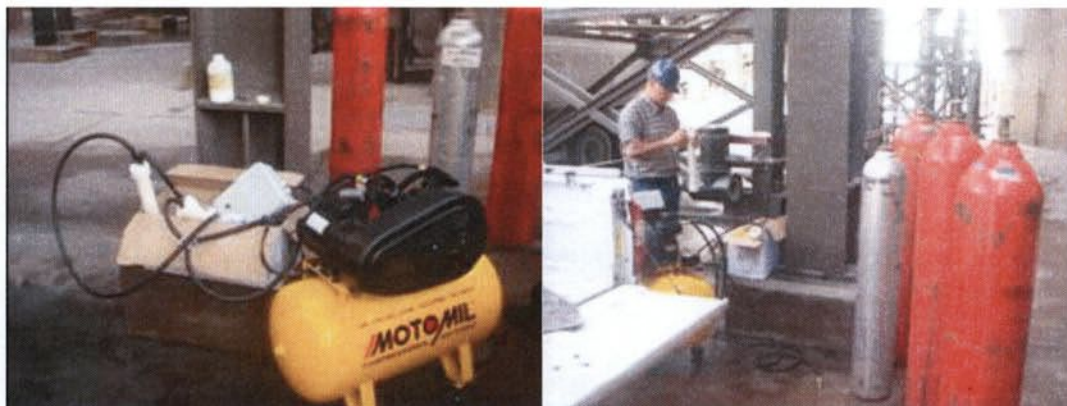
Figura 17: Sistema de captação do gás de combustão – Técnicos do Laboratório Roque L. Zilio e Adriano Arruda Henrard
