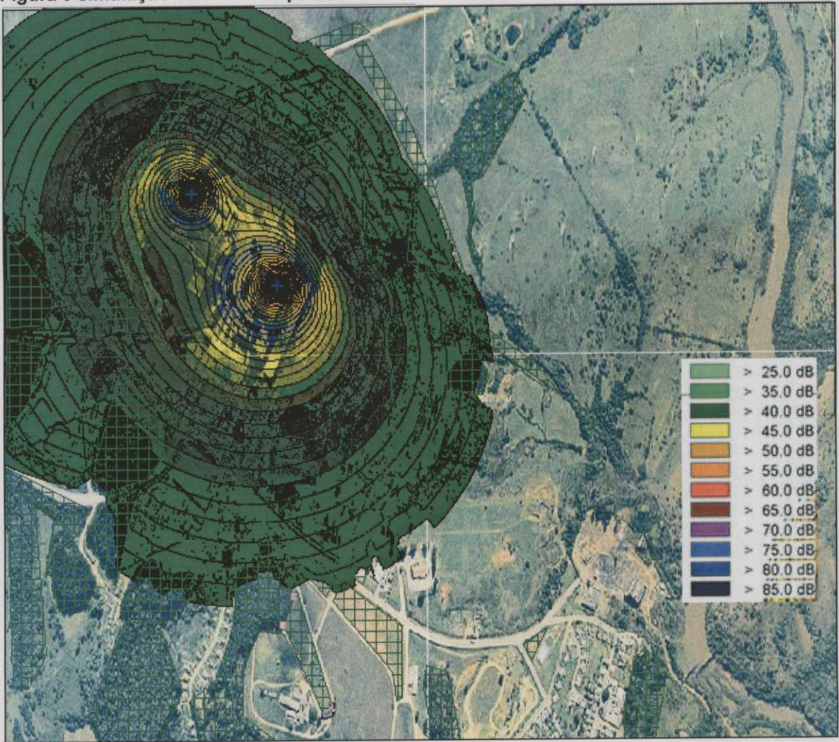
Figura 6 simulação do efeito da pressão sonora da UPME
