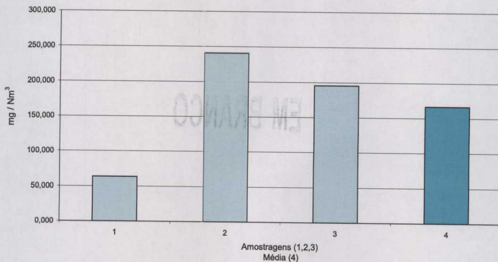
Concentração de H_2SO_4 no efluente
