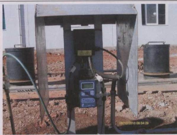
Foto 84 Estação de Tratamento de Efluentes Sanitários – medidor de Turbidez.
