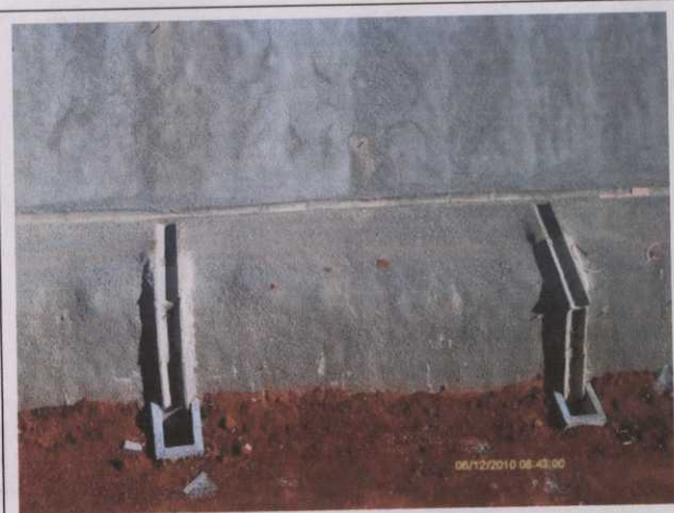
Foto 4 Instalação da drenagem superficial para escoamento das águas pluviais do talude - Concluída
