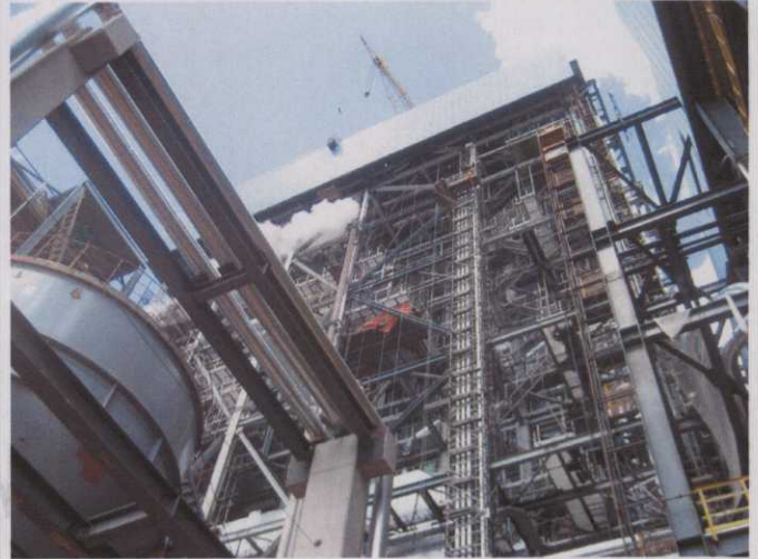
Foto B.12 – Casa da Caldeira, com saída de vapor do balão. Ao lado, o silo de escória.
