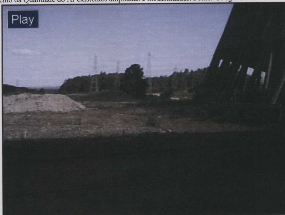
Imagem 3: Provável local da Caldeira Auxiliar para a Fase C, ao lado da Torre de Resfriamento a seco da Fase B, em formato de Torre Hiperbólico.
