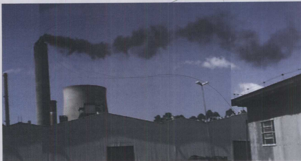
Imagem 1: Dispersão da pluma no dia 26/10/2012.
