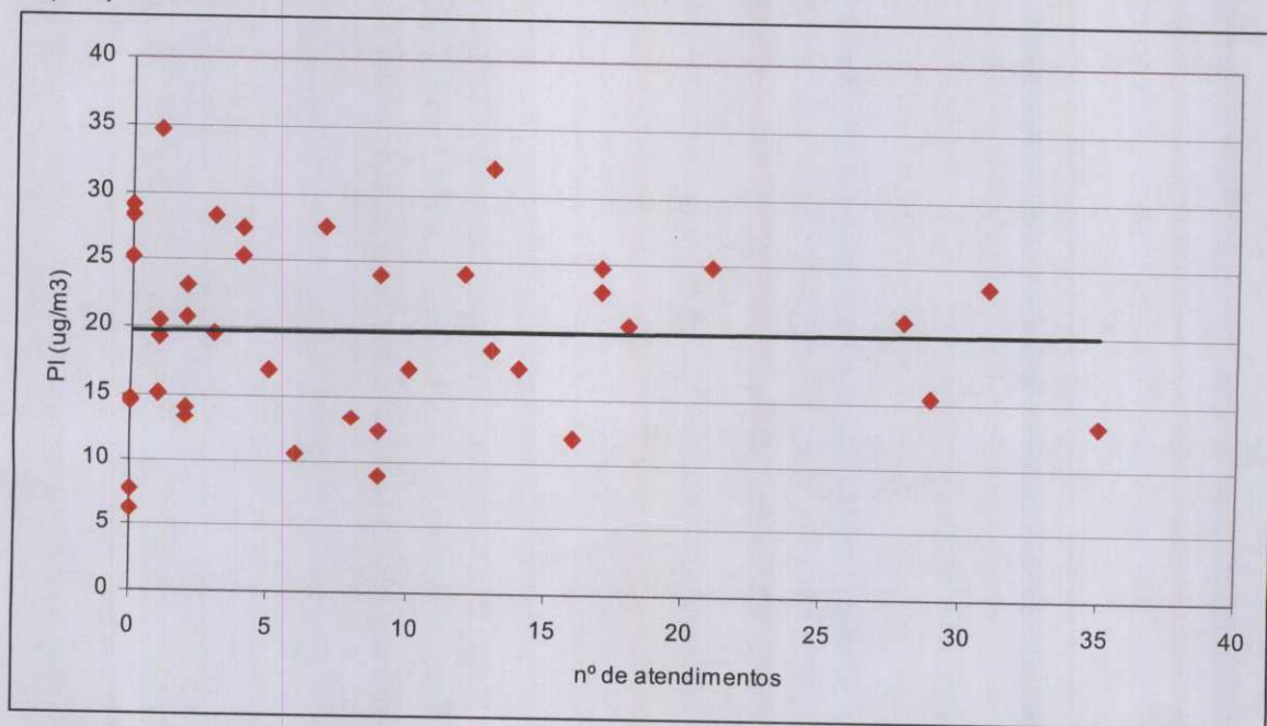
Figura 2. Gráfico de dispersão do número semanal de atendimentos por sintomas respiratórios* em crianças menores de 5 anos nas UBS de Aceguá e a média semanal dos índices de PI da Estação de Aceguá, 01/06/2012 a 15/03/2013.
