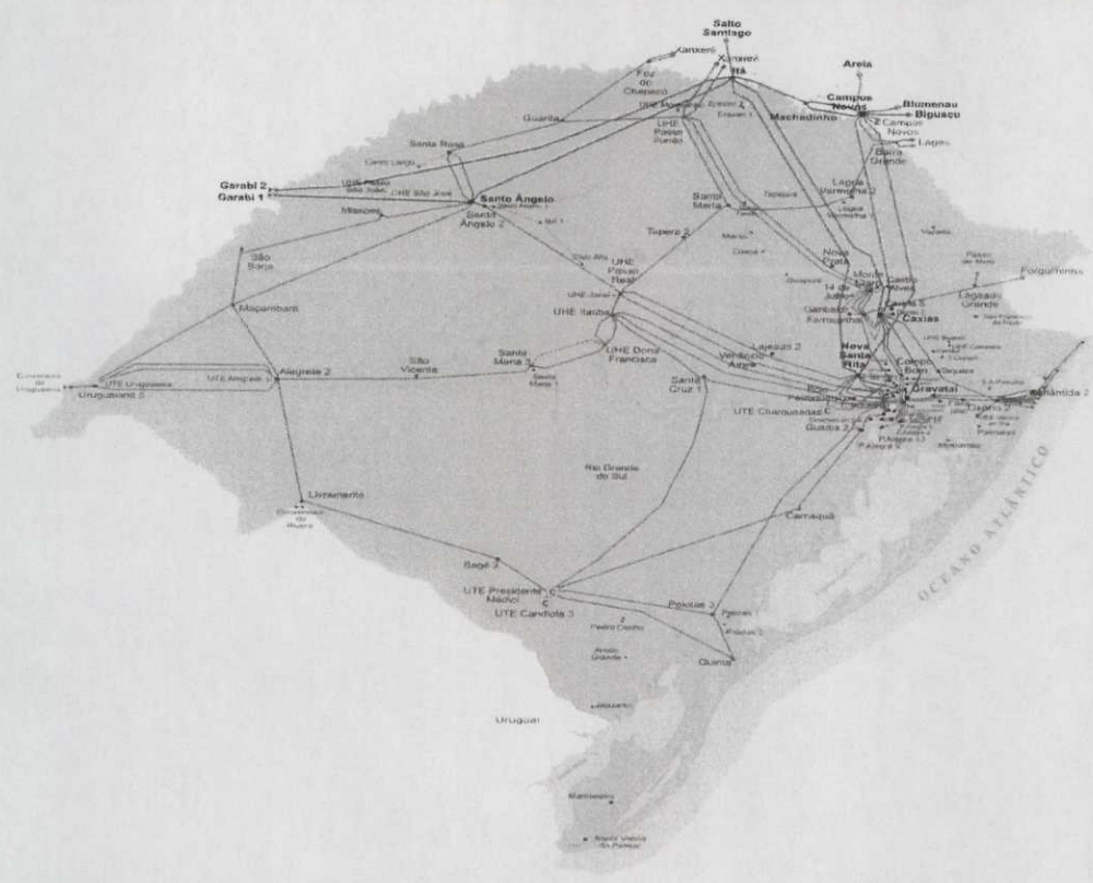
Figura 1-1: Diagrama Eletrogeográfico do Rio Grande do Sul
