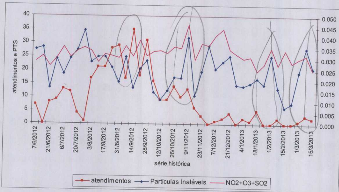
Figura 1. Comparativo entre o número de atendimentos em menores de 5 anos, nas UBS de Aceguá, por sintomas respiratórios*, a média semanal dos índices de PI e a média semanal do total de partículas poluentes (NO 2 , O 3 e SO 2 ), da Estação de Aceguá, 01/06/2012 a 15/03/2013.
