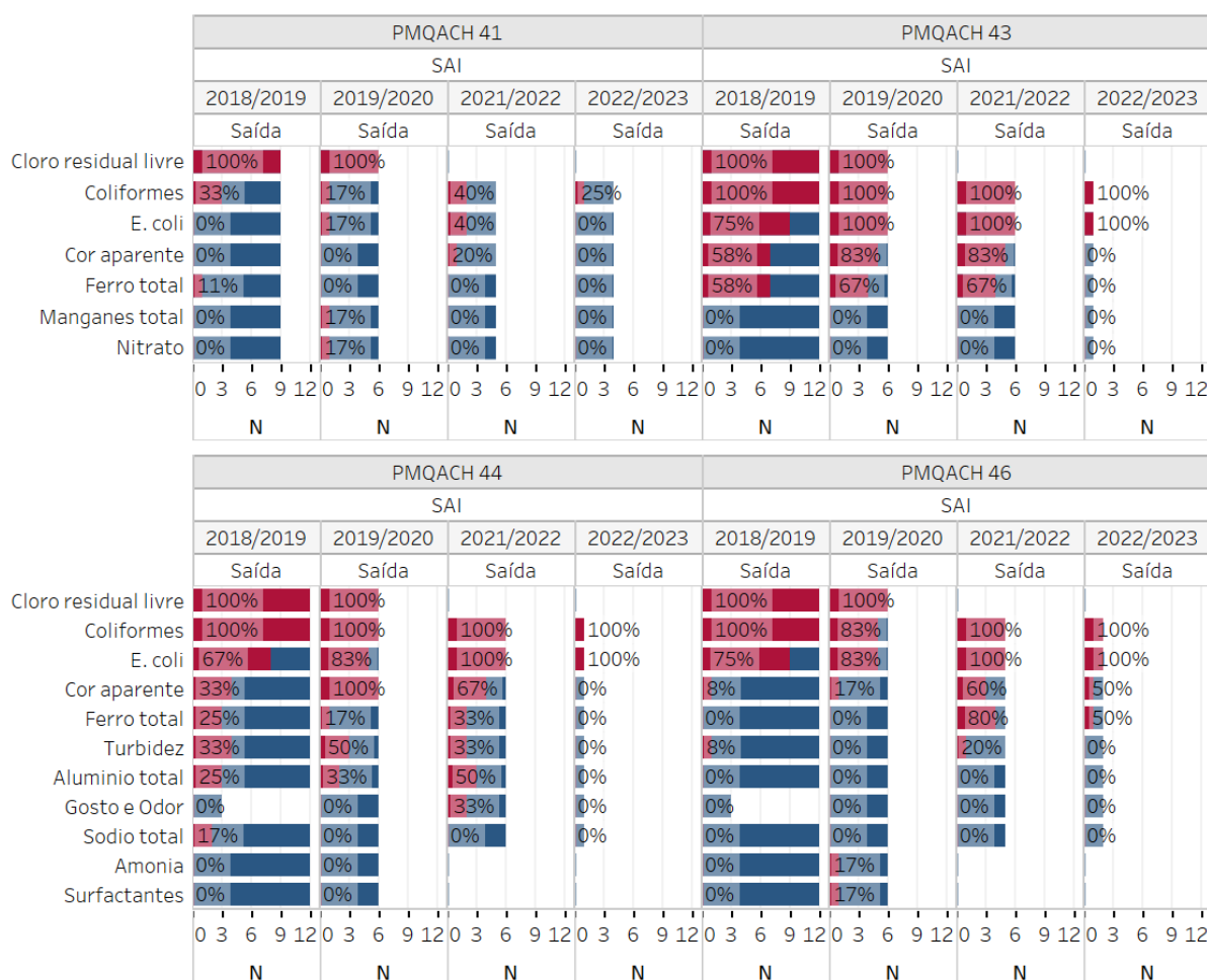
Figura 6-19 - Percentual de violação dos parâmetros monitorados nos pontos PMQACH 41, PMQACH 43, PMQACH 44 e PMQACH 46 localizados no município de Barra Longa-MG, entre setembro/2018 e julho/2023, com base nos limites aplicáveis.
