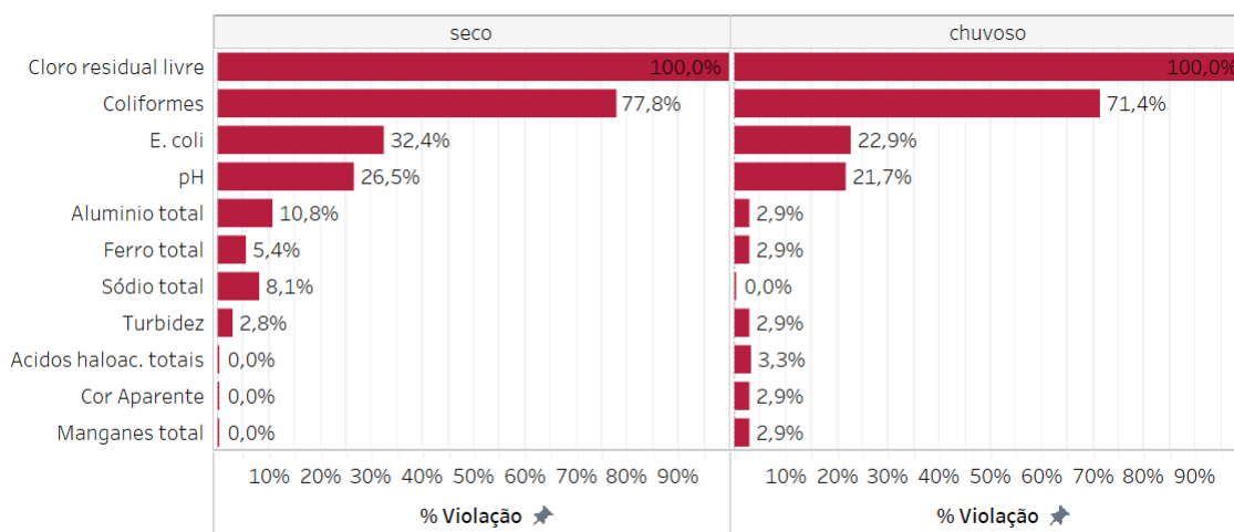
Figura 6-59 - Percentual total de violação para os parâmetros monitorados no ponto sem tratamento do município de São Pedro dos Ferros-MG no período chuvoso (meses de outubro a março) e seco (meses de abril a setembro) entre setembro/2018 e julho/2022 com base nos limites aplicáveis.
