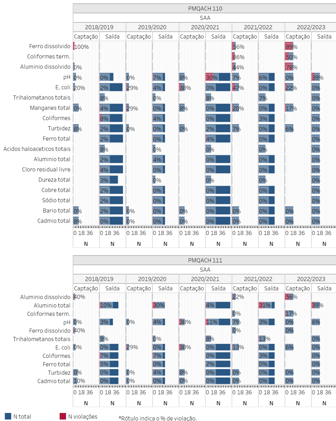
Figura 6-206 - Percentual de violação dos parâmetros monitorados nos pontos PMQACH 110 e PMQACH 111 localizados no município de Colatina-ES, entre setembro/2018 e julho/2023 com base nos limites aplicáveis.
