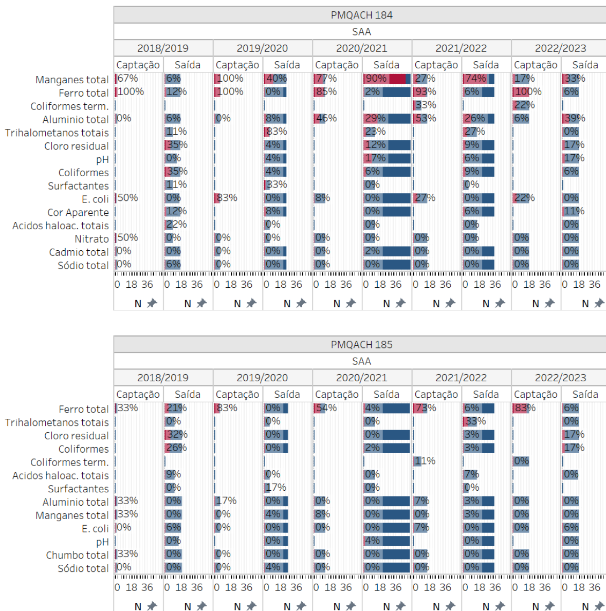
Figura 6-241 - Percentual de violação dos parâmetros monitorados nos pontos PMQACH 184 e PMQACH 185 localizados no município de Linhares-ES, entre setembro/2018 e julho/2023 com base nos limites aplicáveis.
