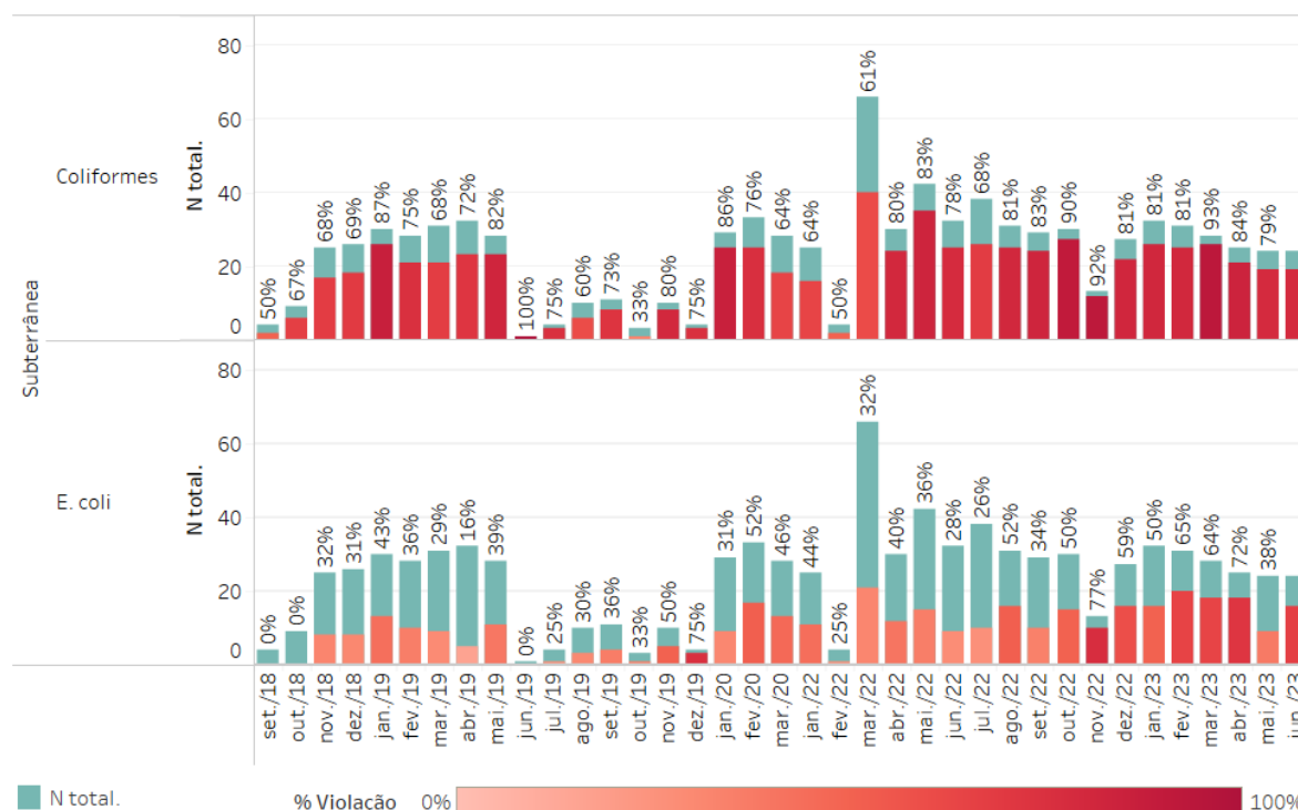
Figura 6-233 - Série histórica dos resultados qualitativos de coliformes totais e E. coli na saída dos pontos sem tratamento, localizados no município de Linhares-ES.
