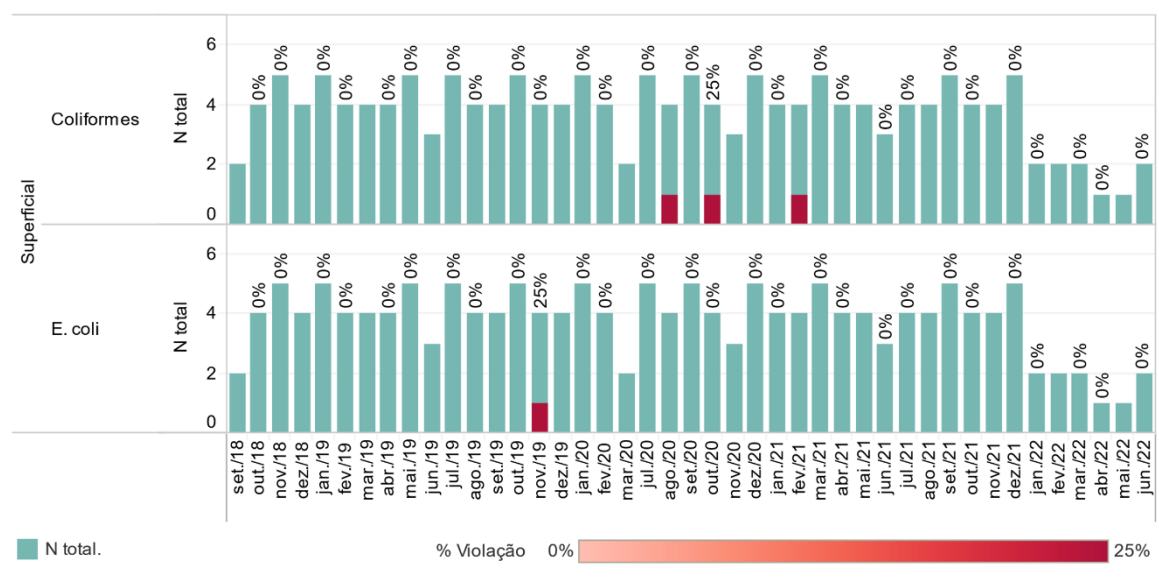
Figura 6-177 - Série histórica dos resultados qualitativos de coliformes totais e E. coli na saída do ponto PMQACH 158, localizado no município de Itueta.
