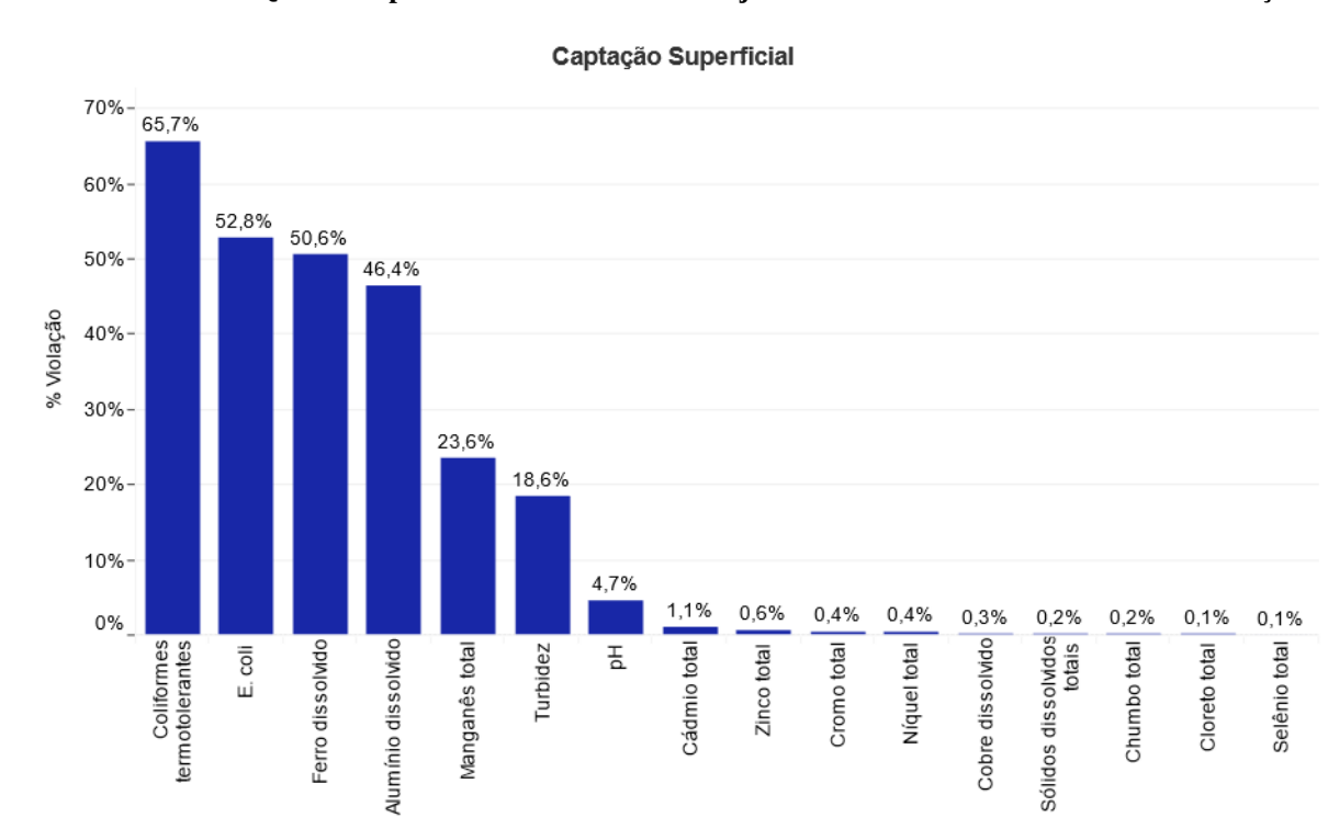
Figura 6-2 - Percentual total de violação dos parâmetros avaliados na captação superficial dos pontos amostrais do PMQACH no período de setembro/2018 a julho/2023. *Rótulos indicam o% de violação.
