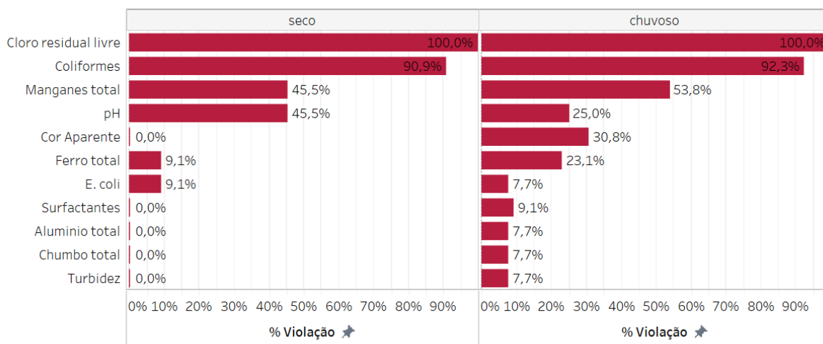
Figura 6-171 - Percentual total de violação para os parâmetros monitorados no município de Itueta-MG no período chuvoso (meses de outubro a março) e seco (meses de abril a setembro) entre setembro/2018 e julho/2023 com base nos limites aplicáveis.
