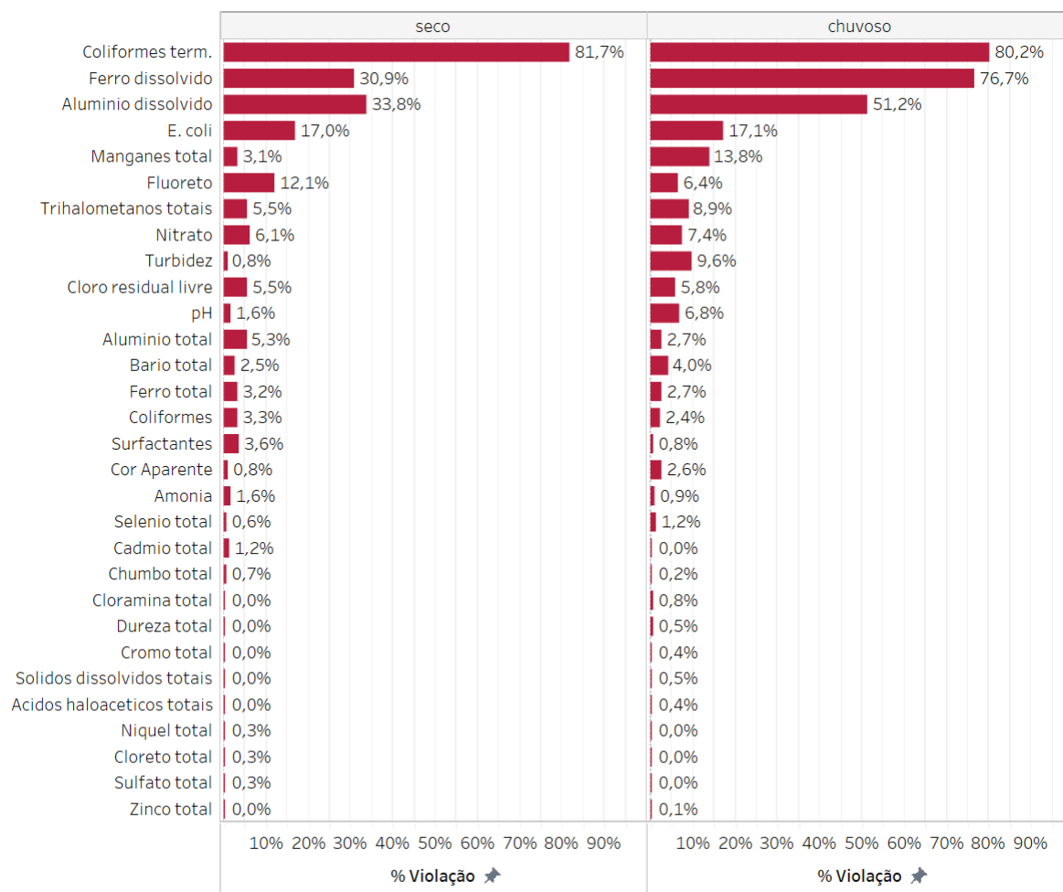
Figura 6-132 - Percentual total de violação para os parâmetros monitorados nos pontos com tratamento no município de Governador Valadares-MG no período chuvoso (meses de outubro a março) e seco (meses de abril a setembro) entre setembro/2018 e julho/2023 com base nos limites aplicáveis.
