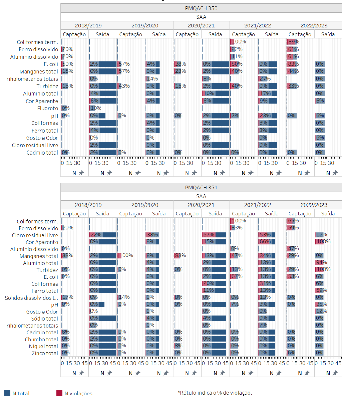
Figura 6-148 - Percentual de violação dos parâmetros monitorados nos pontos PMQACH 350, PMQACH 351 localizados no município de Tumiritinga-MG entre setembro/2018 e julho/2023 com base nos limites aplicáveis.
