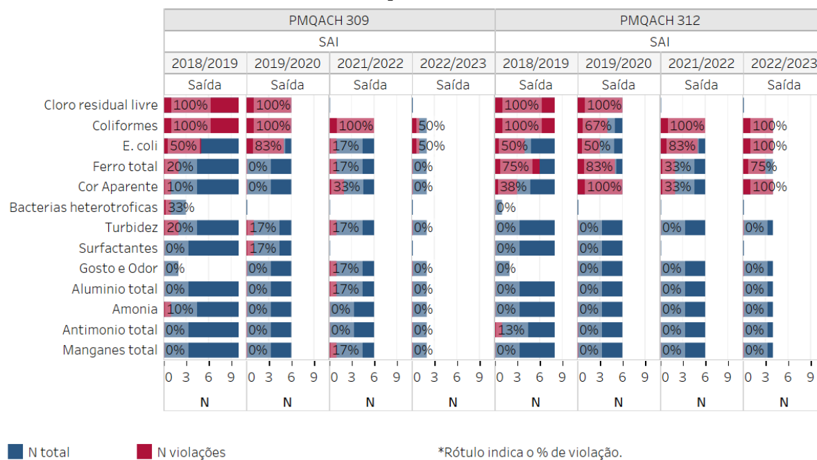
Figura 6-33 - Percentual de violação dos parâmetros monitorados nos pontos PMQACH 309 e PMQACH 312 localizados no município de Rio Doce - MG, entre setembro/2018 e julho/2023, com base nos limites aplicáveis.
