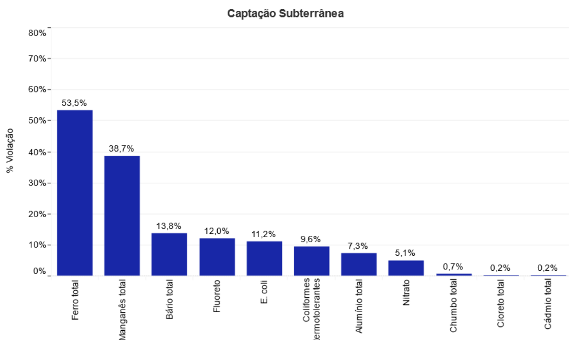
Figura 6-3 - Percentual total de violação dos parâmetros avaliados na captação subterrânea dos pontos amostrais do PMQACH no período de setembro/2018 a julho/2023. *Rótulos indicam o % de violação.
