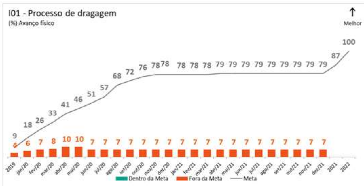
Figura 10 - Gráfico 1. Avanço físico do processo de dragagem. Gráfico Acumulado.
