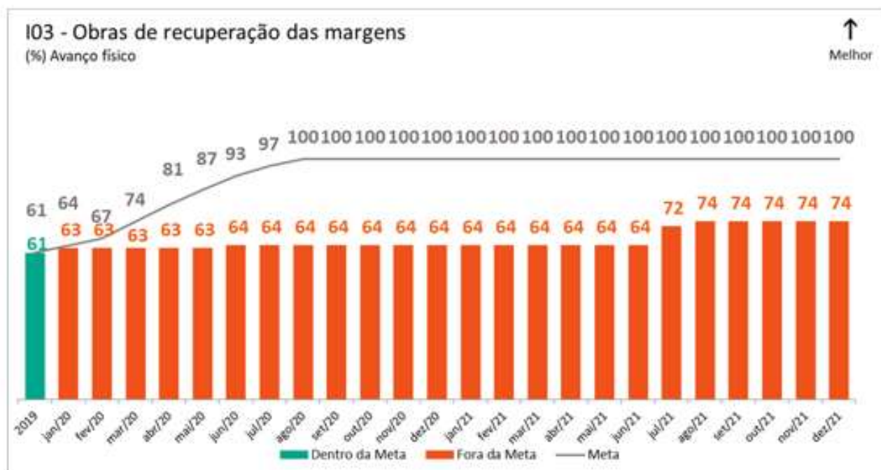
Figura 12 - Gráfico 3. Avanço físico das obras de recuperação das margens. Gráfico Acumulado.
