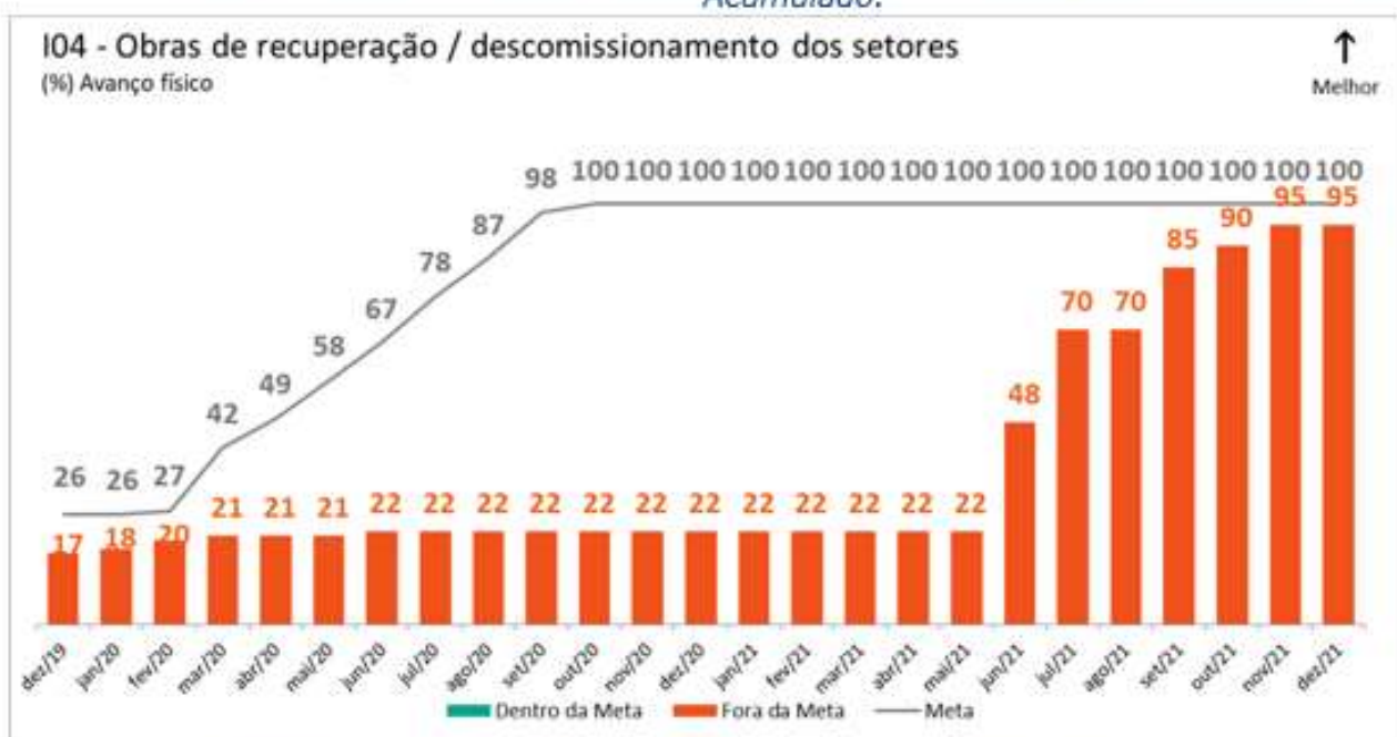
Figura 13 - Gráfico 4. Avanço físico das obras de reabilitação / descomissionamento dos setores. Gráfico Acumulado.
