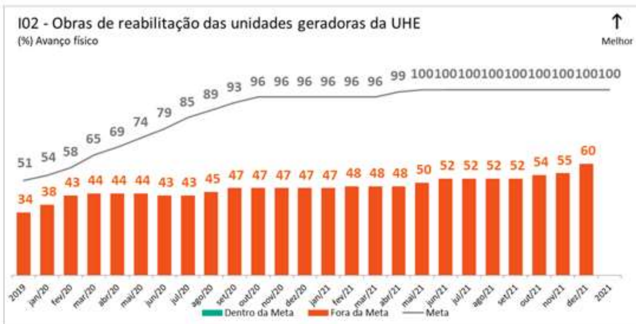
Figura 11 - Gráfico 2. Avanço físico das obras de reabilitação das unidades geradoras da UHE. Gráfico Acumulado.
