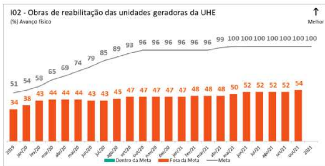
Gráfico 2. Avanço físico das obras de reabilitação das unidades geradoras da UHE. Gráfico Acumulado.
