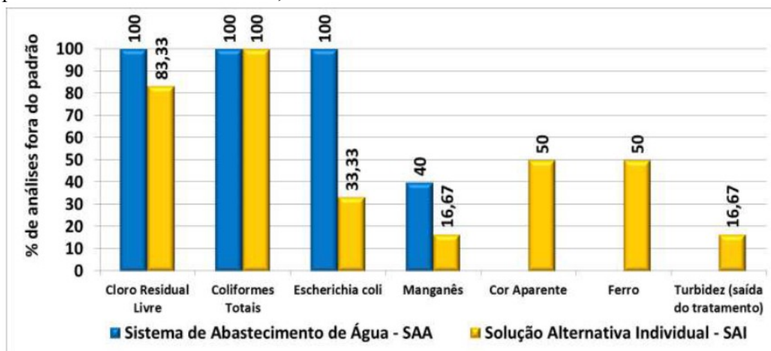
Gráfico 4: Análises de água para o consumo humano com resultados insatisfatórios no período de 18/06/19 - 16/09/19, São José do Goiabal-MG
