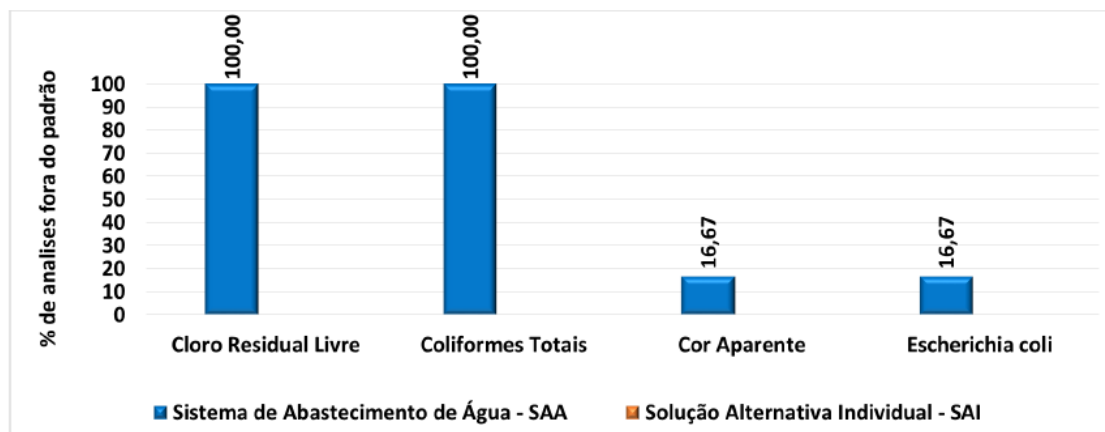
Gráfico 9: Análises de água para o consumo humano com resultados insatisfatórios no período de 17/12/2020 a 16/03/2021, São José do Goiabal-MG
